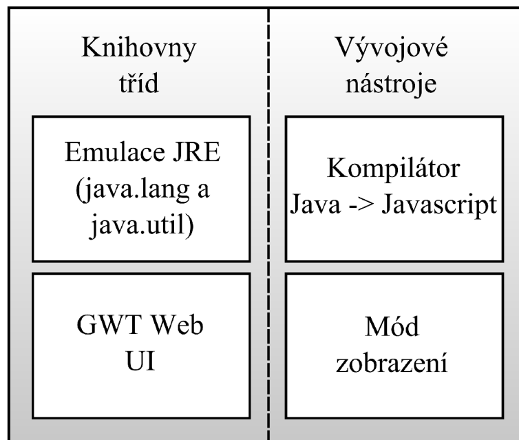
Obr. 3. 3 Struktura GWT
