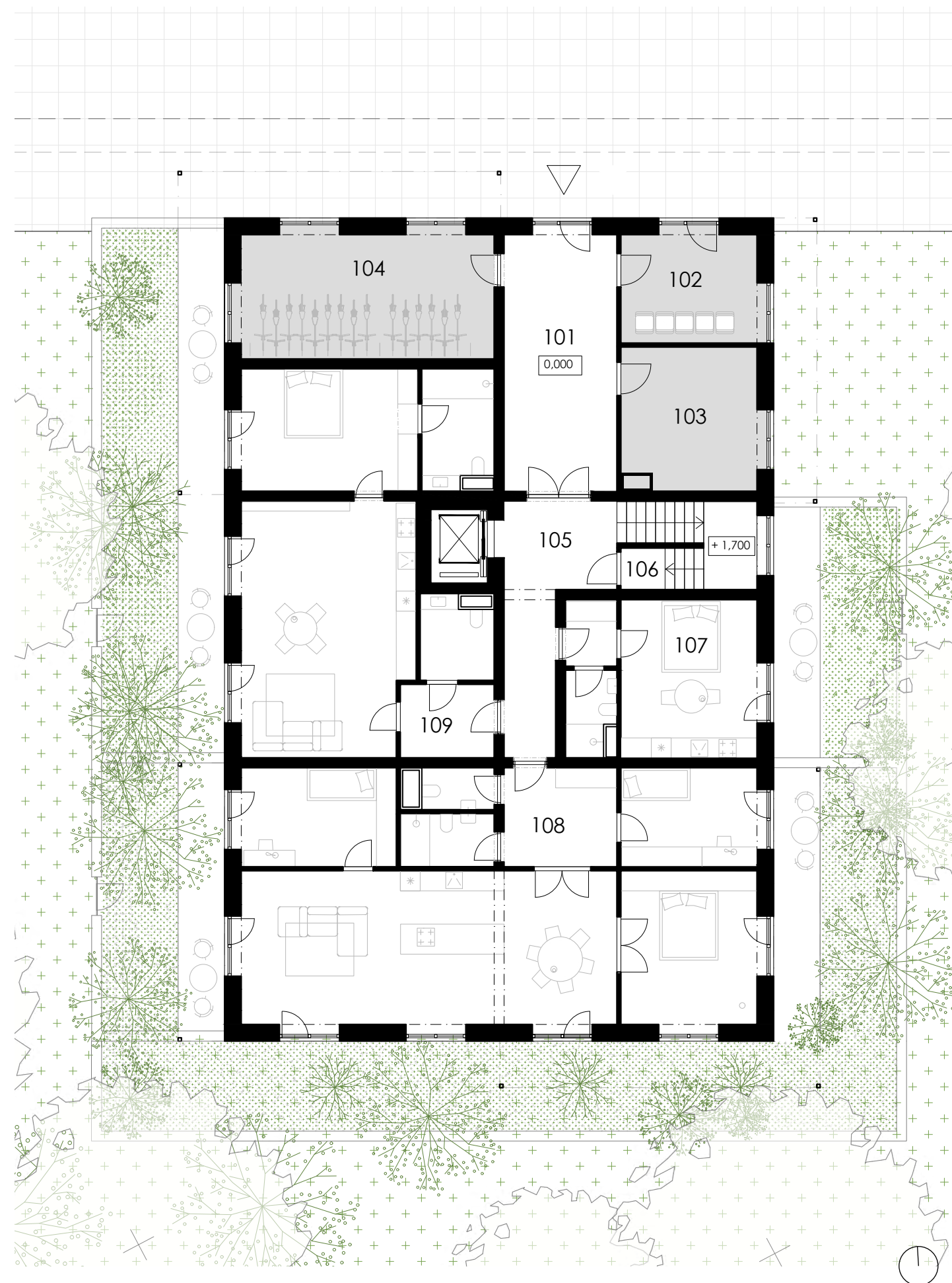
OBJEKT A - PŮDORYS 1NP 1:150
