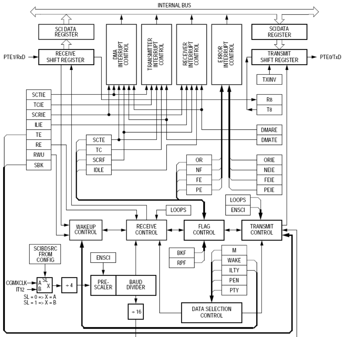
Obrázek 3.1: Blokové schéma modulu SCI
