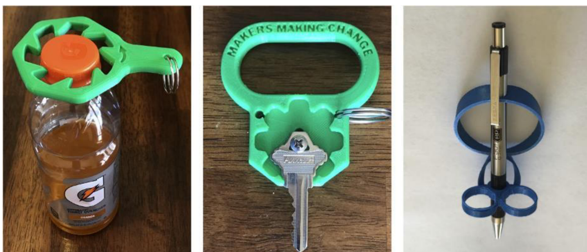
Obrázek 25 Vytisknuté kompenzační pomůcky pro otevírání plastových lahví, manipulaci s klíči a psaní pro osobu s revmatoidní artritidou (Janson et al., 2020, s. 165–166)
