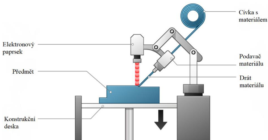
Obrázek 5 DED tiskárna
