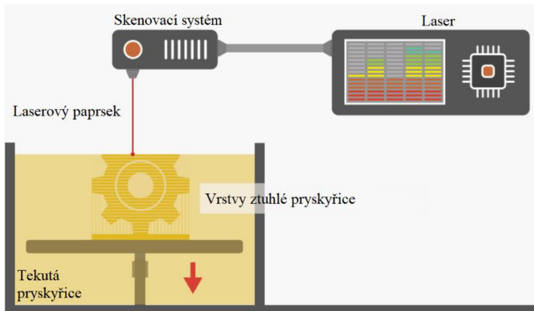
Obrázek 1 SLA tiskárna (převzato z: https://3dprintingindustry.com/3d-printing-basics-free-beginners-guide/#04-processes )
