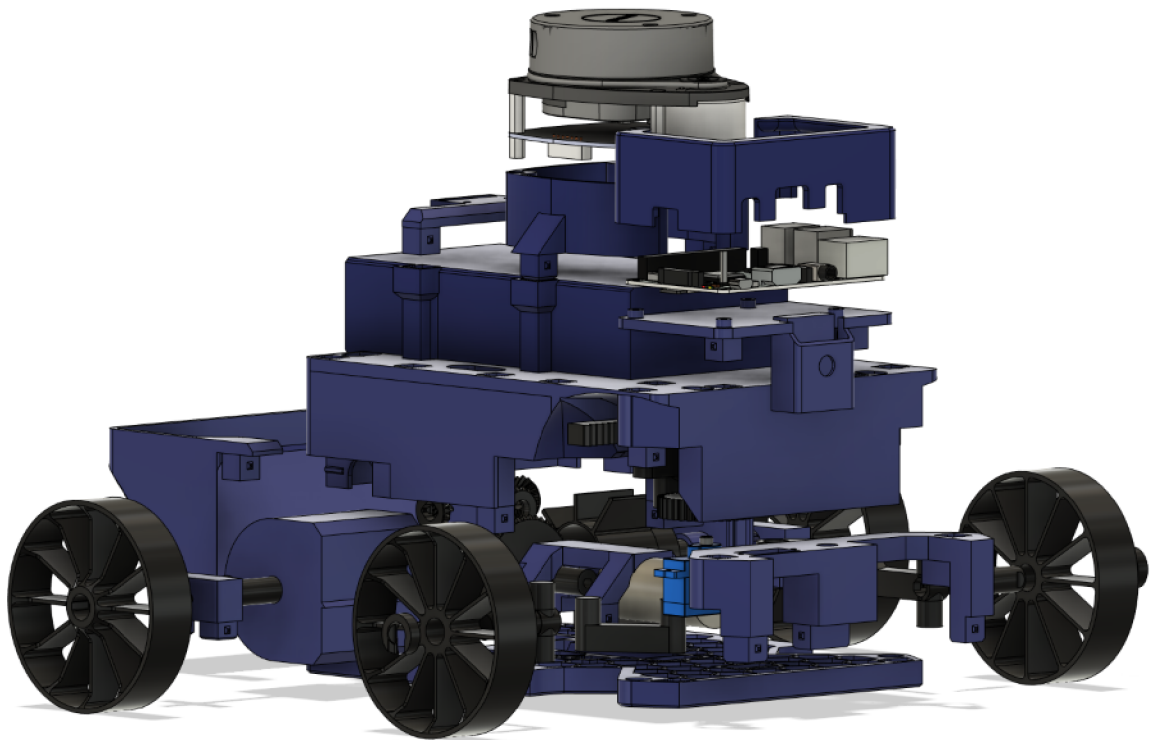
Obrázek 5.6: Rozložené vozidlo
