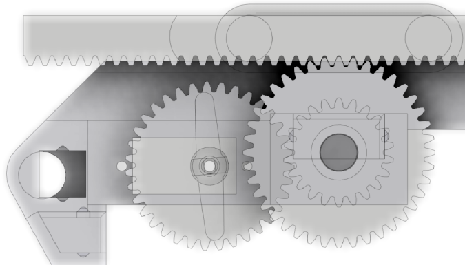
Obrázek 5.19: Převody serva a ozubeného hřebenu
