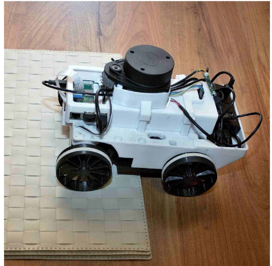
(d) Měření schopnosti překonávat schod
