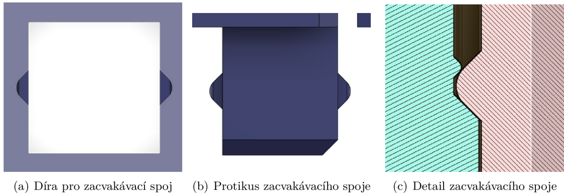
Obrázek 5.7: Zacvakávací spoj
