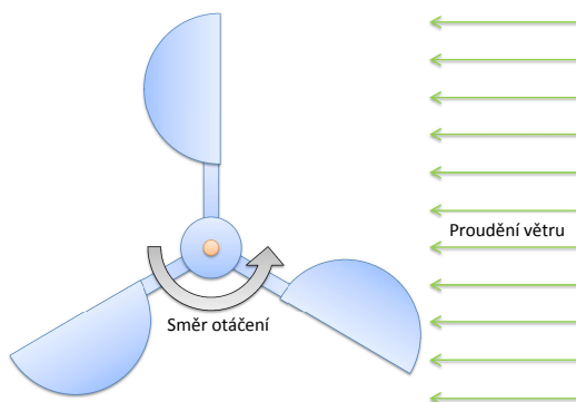
Obrázek 2.14: Mechanické schéma lopatkového anemometru
