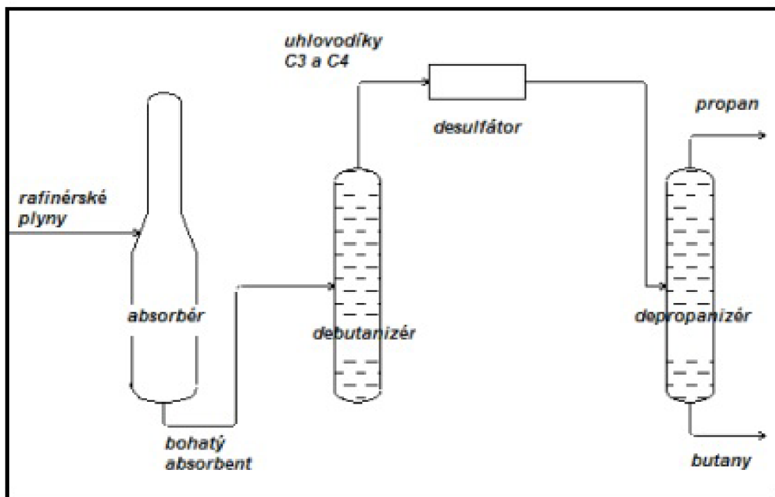
Obrázek 3.11: Výroba LPG ze surové ropy, (Štěrba a Kryžický, 2002)
