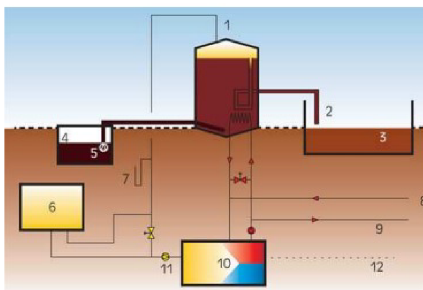
Obrázek 3.22: Schéma bioplynové stanice, (Ekowatt.cz, 2007)
