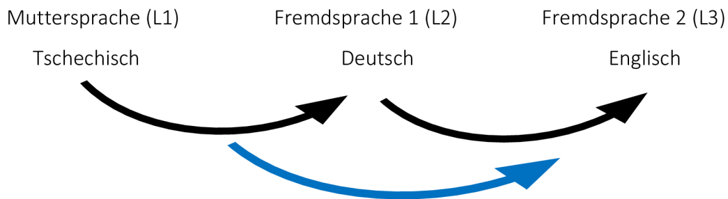
Abbildung 3: Proaktive Interferenz
