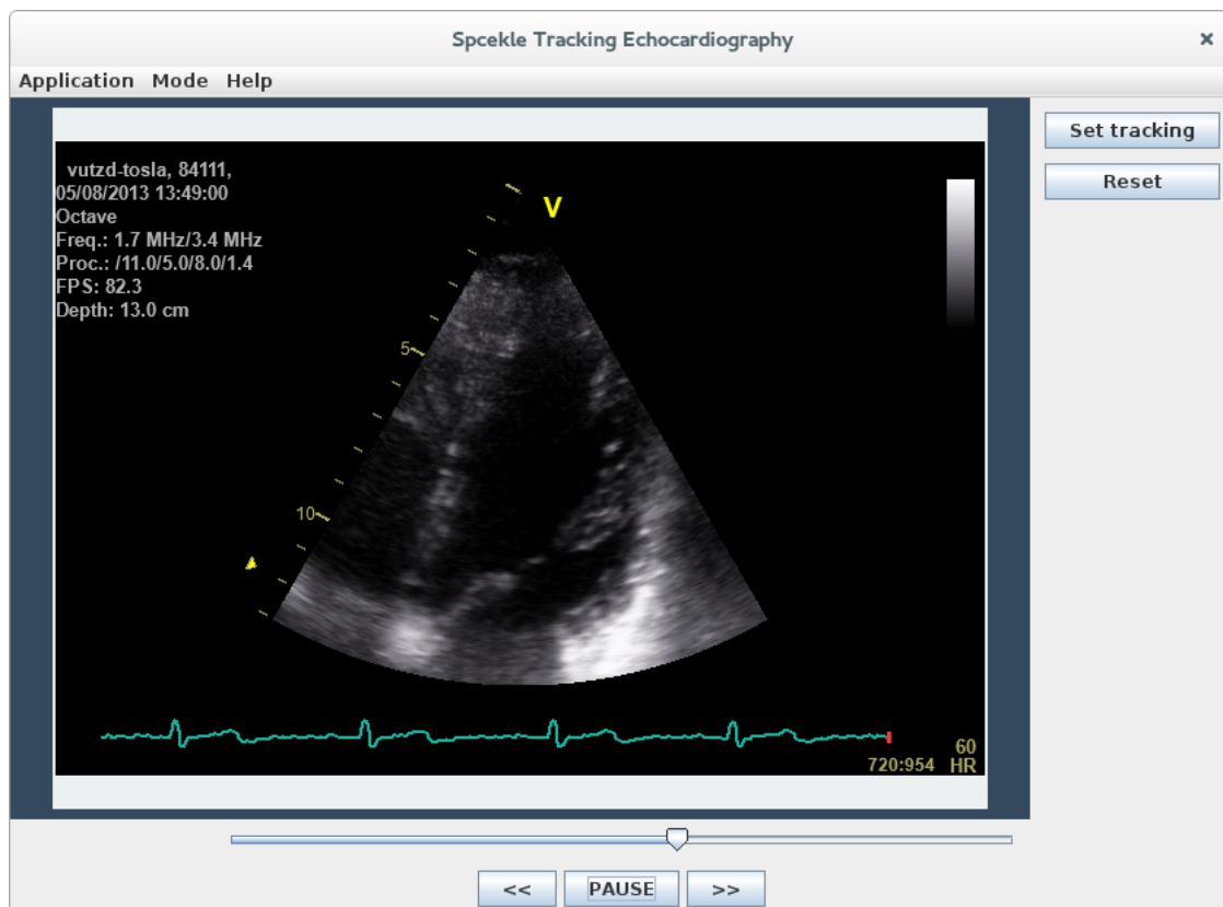
Obrázek 5.2: Prehrávanie videa.
