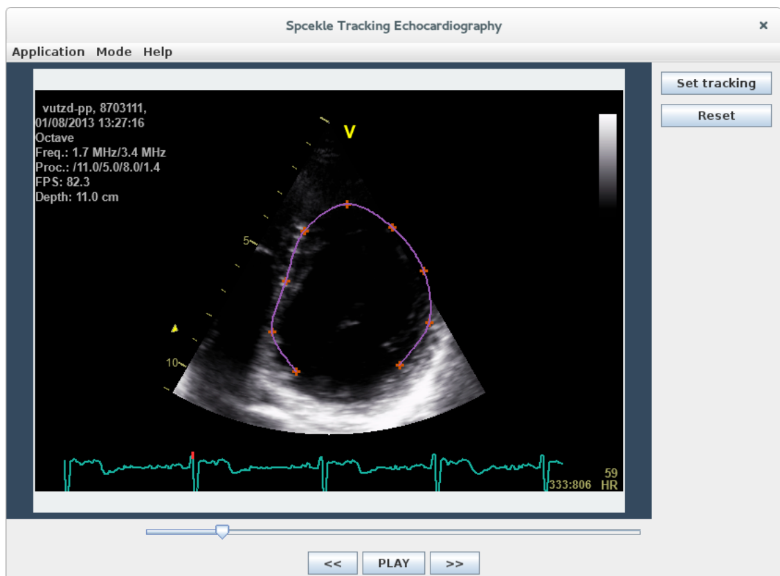
Obrázek 5.4: Sledovanie tvaru.
