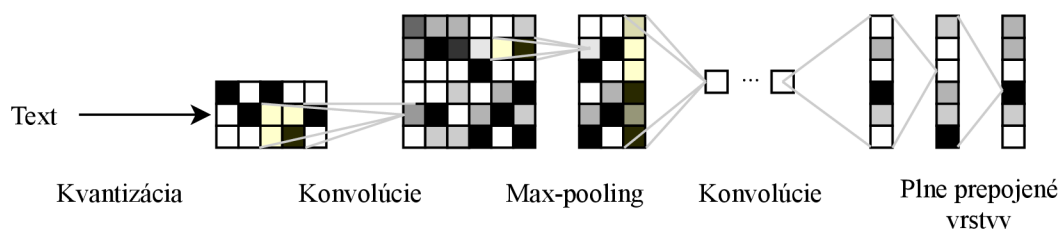
Obr. 5.6: Model konvolučnej siete na úrovni charakterov [37]
