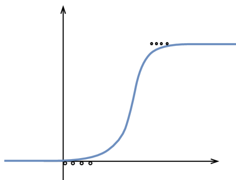
Obr. 3.1: Logistická regresia
