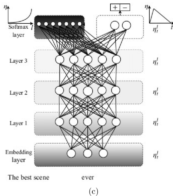
Obr. 5.8: ULMFiT architektúra modelu pre jednotlivé fázy tréovania: a) predtrénovanie jazykového modelu na všeobecnej dátovej sade, b) diskriminačný fine-tuning modelu na dátovej sade z riešenej domény, c) tréovanie klasifikátora, prechod bielej farby do čiernej znázorňuje postupné umožnenie ladenia [15]
