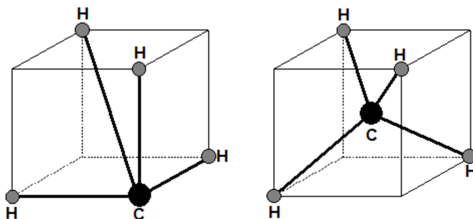
Obr. 5: Porovnání tvaru molekuly \text{CH}_4 vypočteného pomocí teorie MO (vlevo) a stanoveného experimentálně (vpravo). Vzato z (Čídlková, Mokrý, and Valová 2008).
