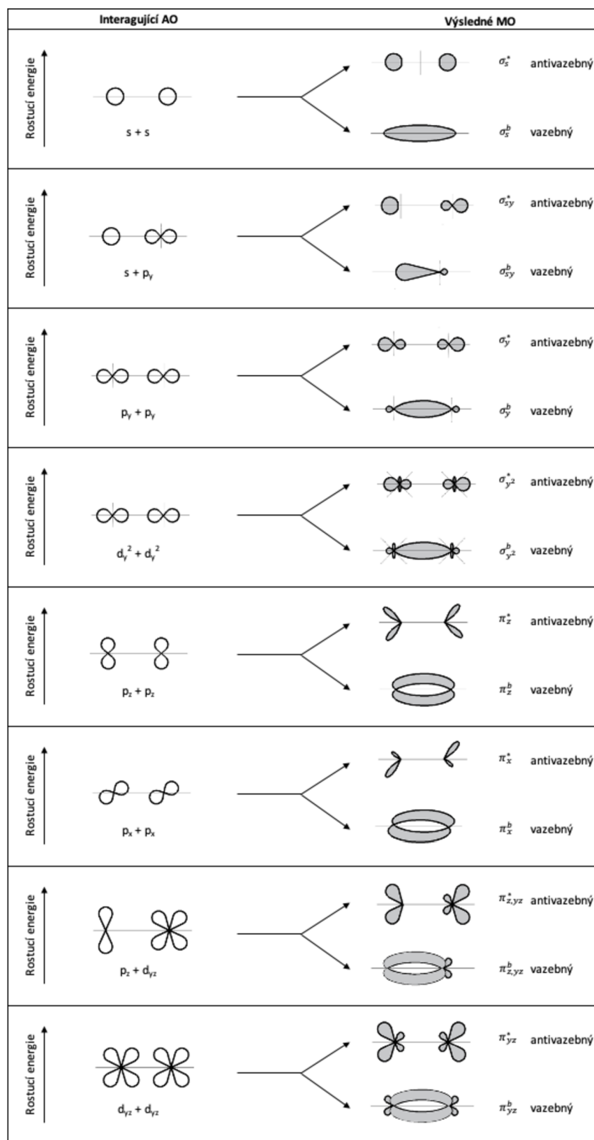
Obr. 4: Znáornění interagujících atomových orbitalů (AO) a molekulových orbitalů (MO)vzniklých jejich překryvem. Upraveno podle (Cídllová, Mokrá, and Valová 2008).
