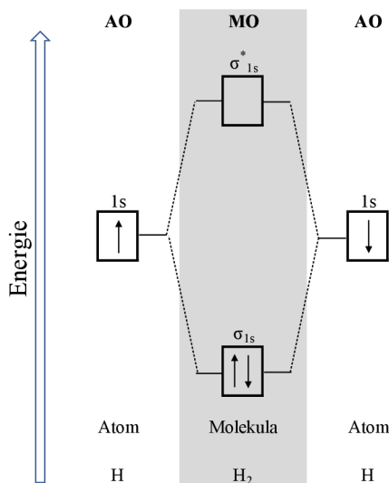
Obr. 3: Diagram MO molekuly H 2 . Převzato z (Cídllová, Mokrá, and Valová 2008).
