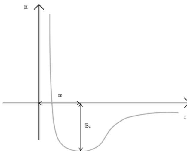
Obr. 1: Graf vzajemneho siloveho psobenı dvou atomu v zavislosti na vzdalenosti mezi nimi, kde E je potencialnı energie soustavy dvou atomu, r je vzdalenosti mezi jadry atomu, r_0 je delka chemicke vazby a E_d je disocianı energie. Prevzato z (Cıdllova, Mokra, and Valova 2008).
