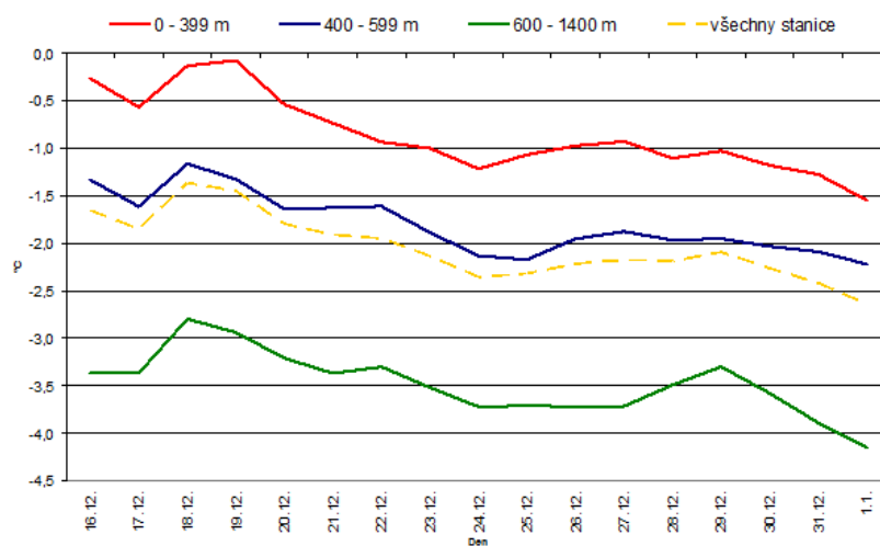
Obr. 1: Průběh průměrné denní teploty vzduchu v období 16. 12. až 1. 1. v letech 1961-2008 pro stanice v různých výškových pásmech (0-399 m, 400-599 m, 600-1400 m), zdroj: Vánoční obleva v Česku - fakt nebo mýtus? Meteorologické zprávy (2009), Škáchová, Žák
