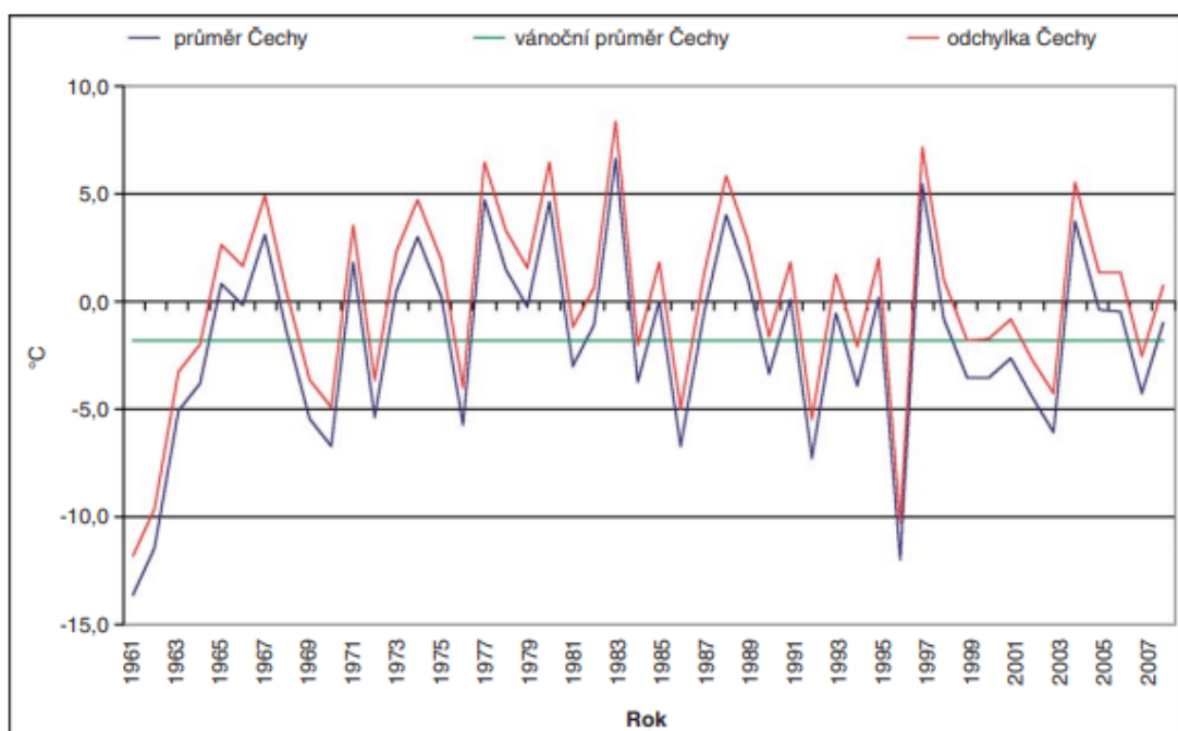
Obr. 1 Průměrná teplota vzduchu o vánočních svátcích v chronologickém pořadí od roku 1961 do 2008 vzhledem k dlouhodobému průměru (1961–2000) v době Vánoc a odchylky jednotlivých let od tohoto dlouhodobého průměru pro Čechy.
