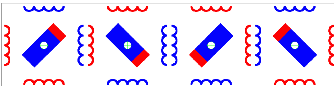
Obr. 3.5: Bipolární dvoufázové řízení krokového motoru s plným krokem
