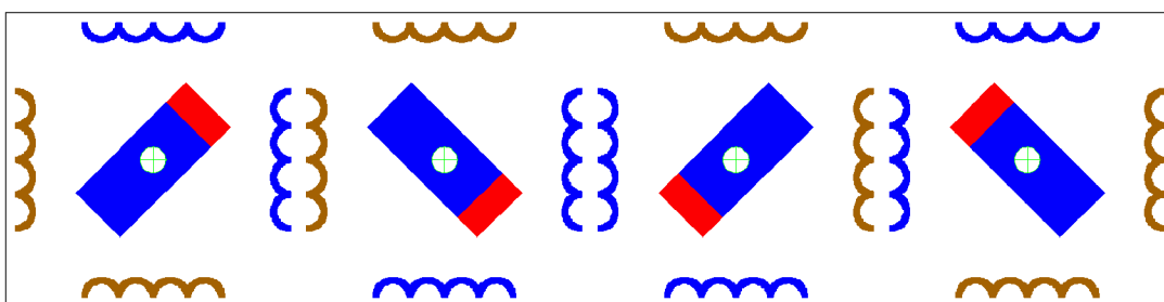
Obr. 3.4: Unipolární dvoufázové řízení krokového motoru s plným krokem
