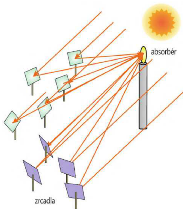
Obr. 1.7: Koncentrátorový systém s centrální věží
