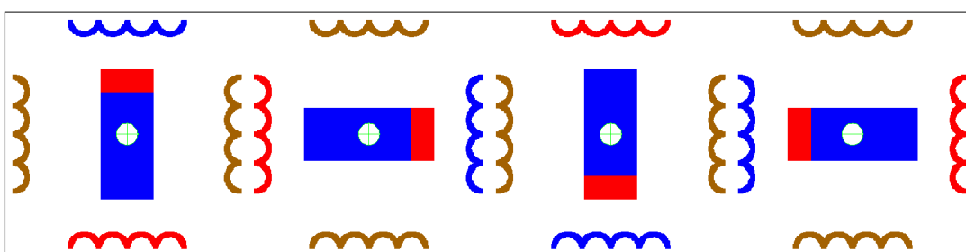
Obr. 3.3: Bipolární jednofázové řízení krokového motoru s plným krokem
