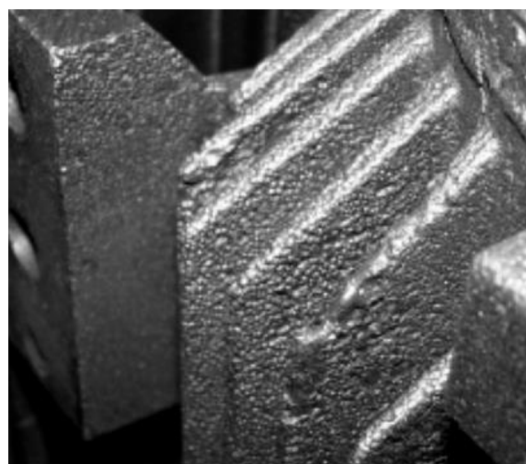
Obr. 32 Řídký povrch [2]
