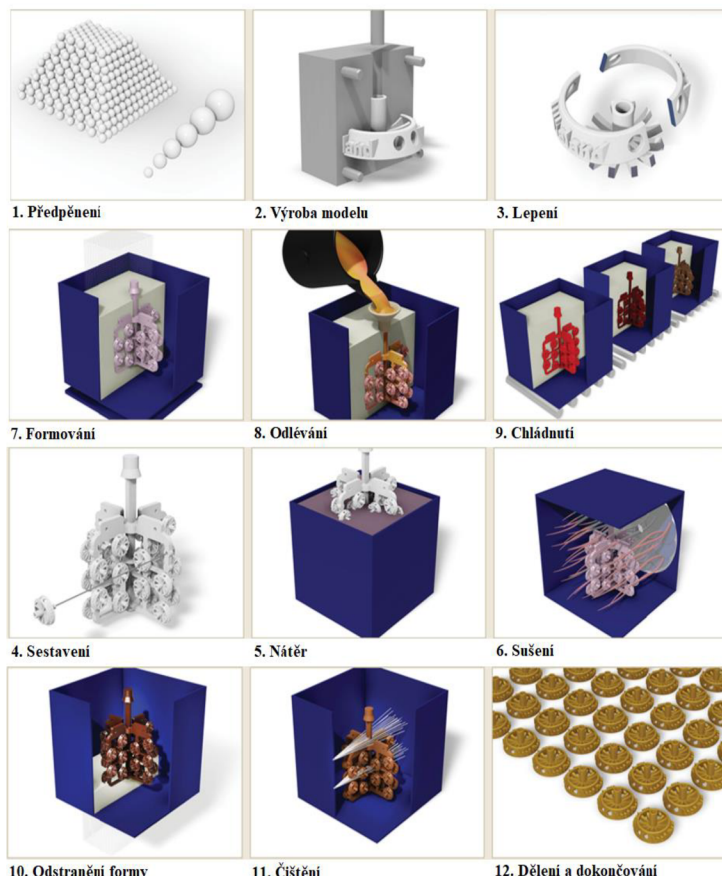
Obr. 2 Schéma technologie [15]
