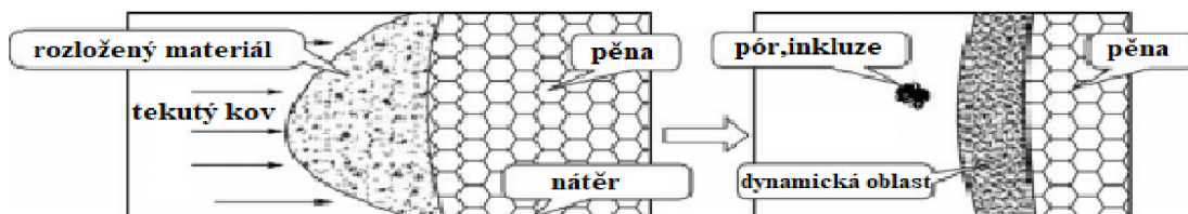
Obr. 27 Schéma postupujícího tekutého kovu [5]
