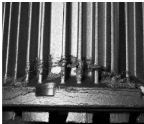
Obr. 31 Utržení odlitku [2]
