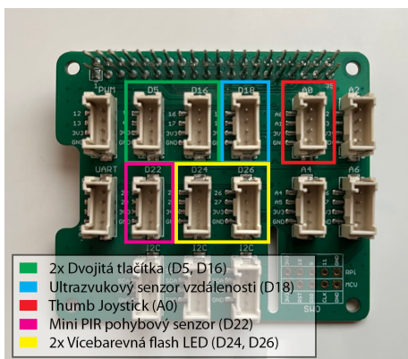
Obrázek 3.15: Umístění zapojení modulů do Grove Base HAT
