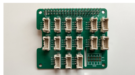
Obrázek 3.4: Grove Base HAT
