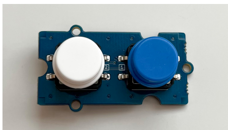
Obrázek 3.7: Grove - Dvojité tlačítko
