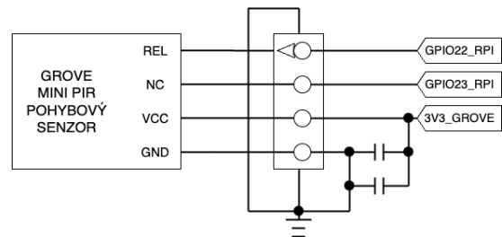
Obrázek 3.12: Grove - Mini PIR pohybový senzor - diagram [10]
