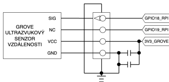
Obrázek 3.10: Grove - ultrazvukový senzor vzdálenosti - diagram [10]
