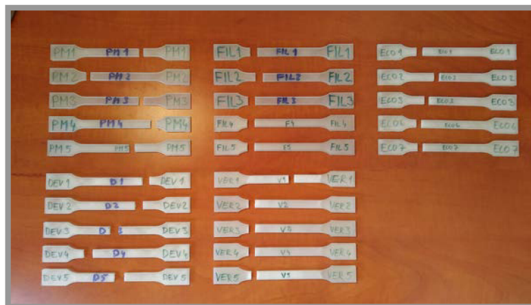
Obr. 21 Skúšobné telesá po ukončení testov
