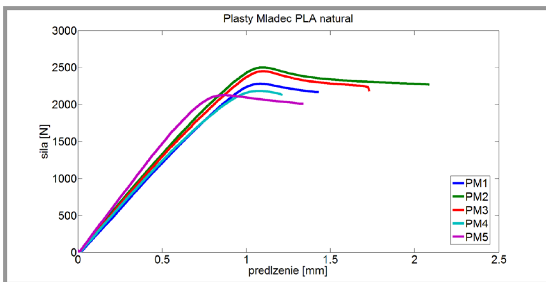
Obr. 27 Ťahové krivky Plasty Mladeč
