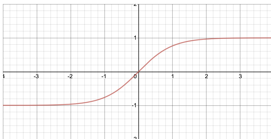
Obrázek 3.3: Hyperbolický tangens.
