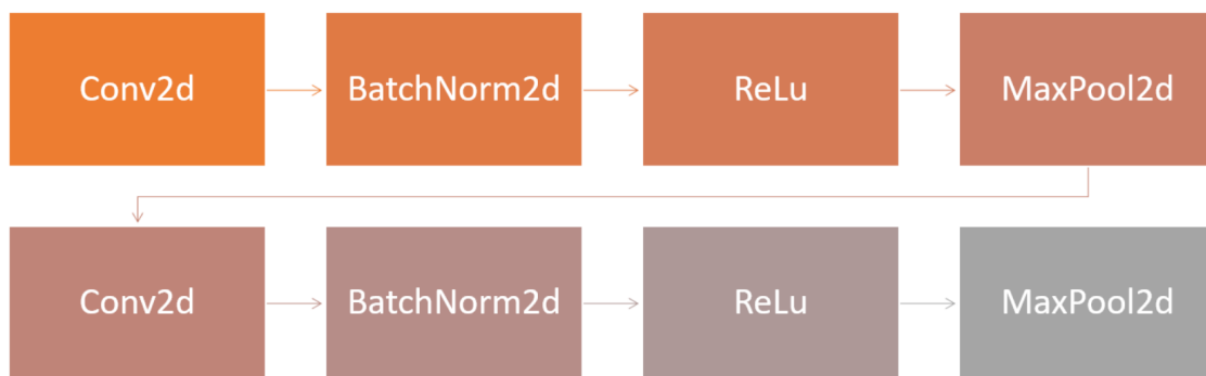
Obrázek 5.0: VGG blok.
