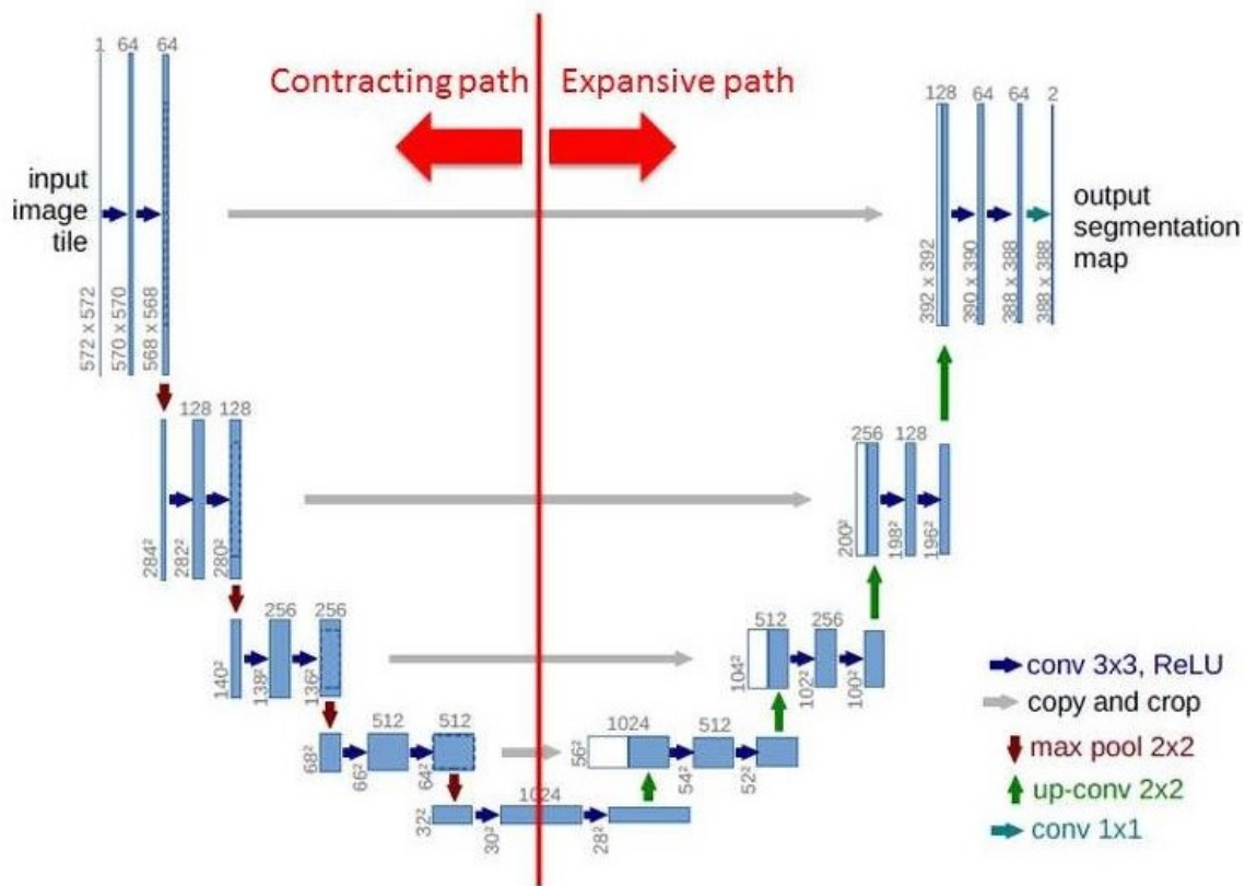
Obrázek 3.7: UNet architektura [15].
