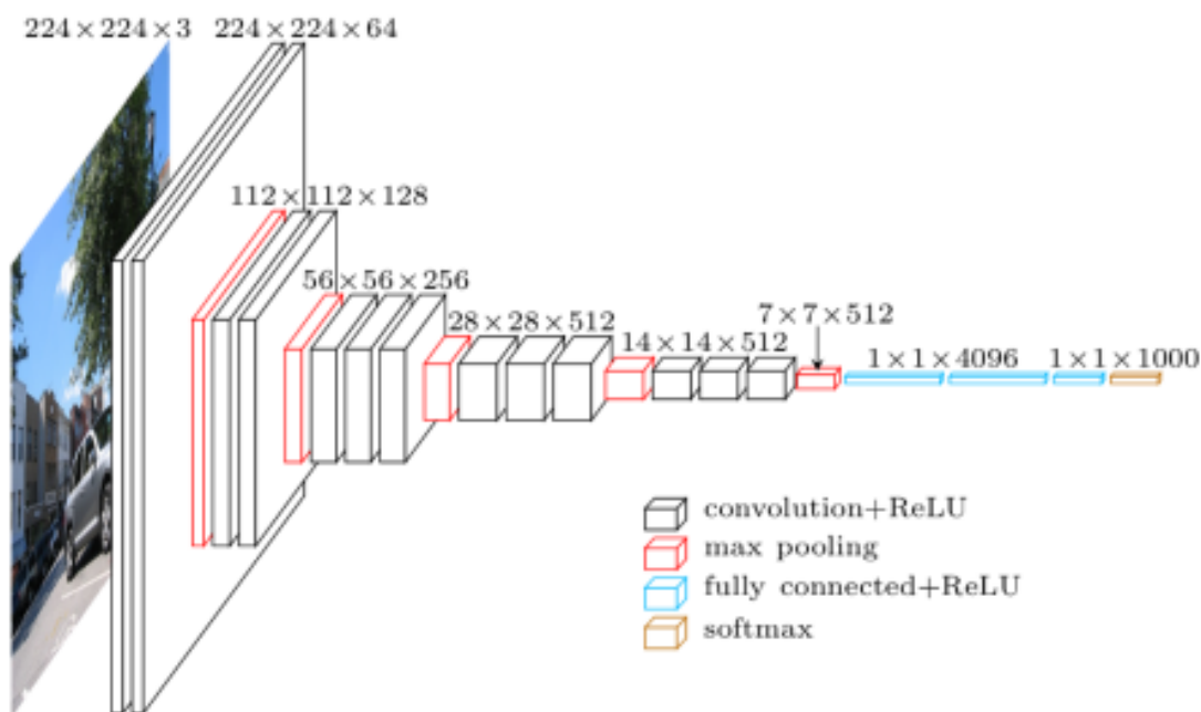
Obrázek 3.6: VGG architektura [2].
