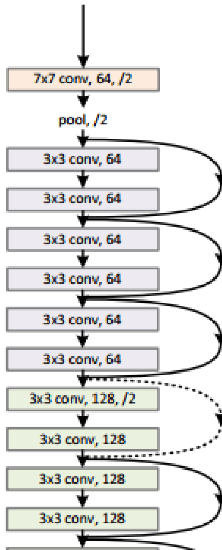
Obrázek 3.8: ResNet architektura [1].
