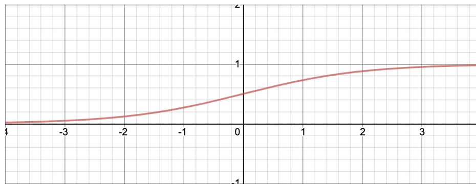
Obrázek 3.2: Sigmoida.
