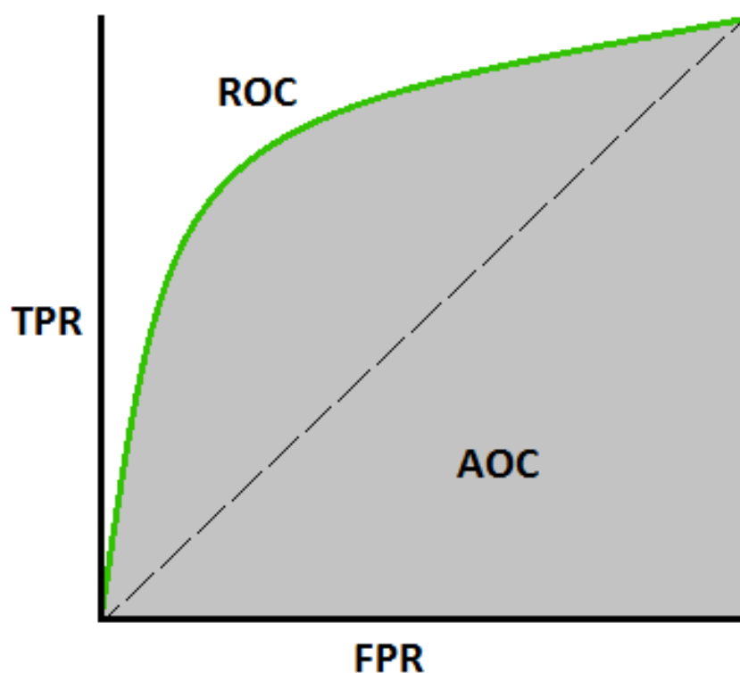
Obrázek 3.5: AUC-ROC křivka.
