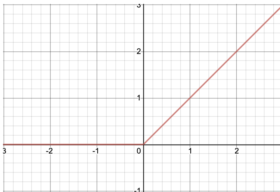
Obrázek 3.1: ReLU.
