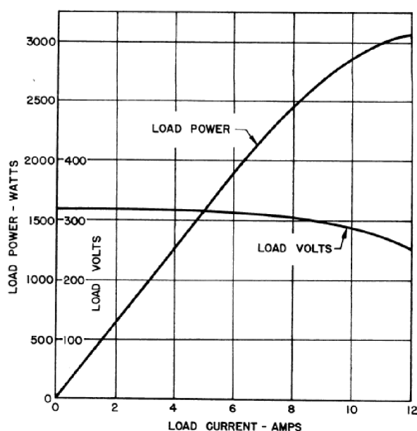
Obrázok 1.3 Závislosť výstupného výkonu a napätia na výstupnom prúde [2]
