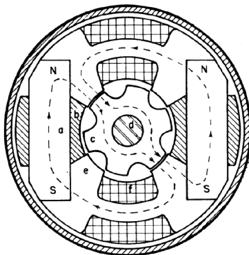
Obrázok 1.2 Prierez konštrukciou navrhovaného alternátora [2]
