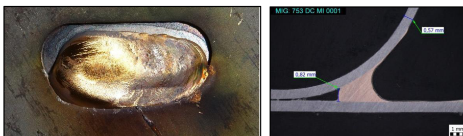
Obr. 9 – MIG pájení
