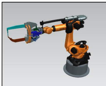
Obr. 42 – Namontované svařovací kleště
