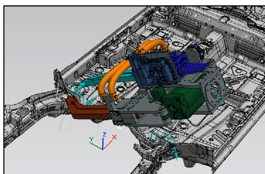
Obr. 38 – Výsledná matice
