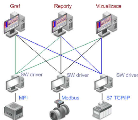
Obrázek 2.1: Komunikace zařízení bez použití technologie OPC [2]
