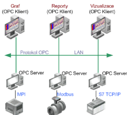
Obrázek 2.2: Použití technologie OPC [2]
