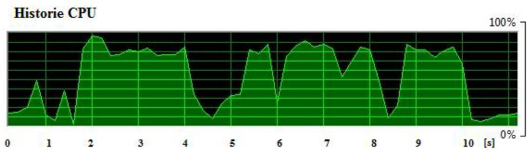
Obrázek 6.6: Zatížení CPU - 3000 tagů (OPC DeltaLogic)
