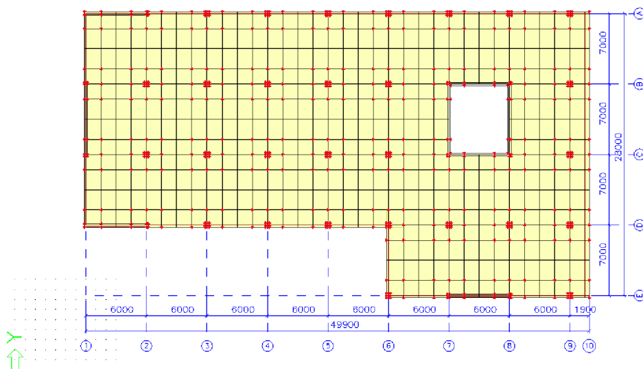
Obr. 1 Půdorys objektu
