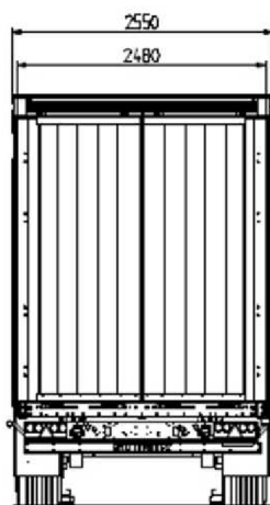
Obrázek 3.5: Šířka návěsu SCHMITZ CARGOBULL S.CS 24/L
