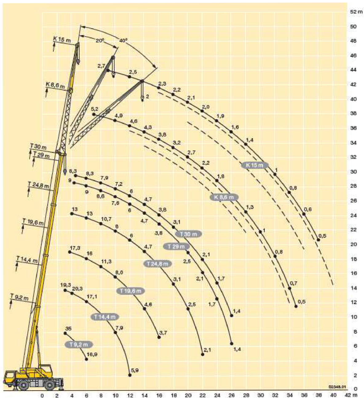
Obrázek 3.16: Zátěžový diagram autojeřábu LIEBHERR LTM 1030-2.1
