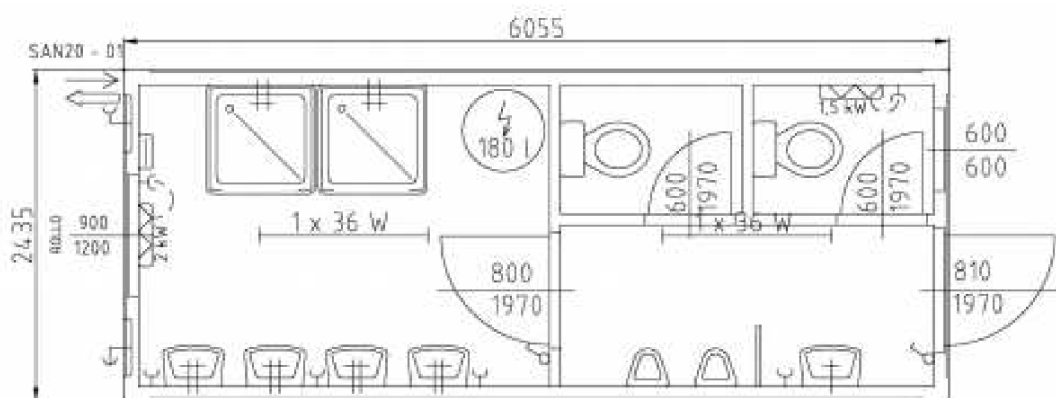
Obrázek 2.3: Půdorysné schéma sanitární buňky SAN20-01
