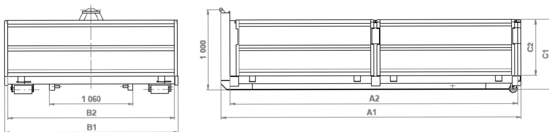
Obrázek 3.19: Délkové parametry valníkového kontejneru
