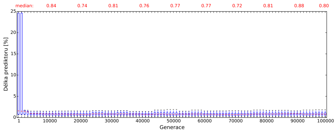
(b) 50% impulzní náhodný šum
