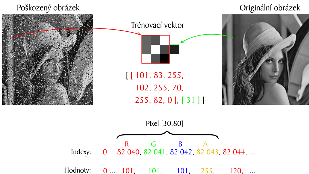
Obrázek 4.1: Ukázka vytvoření jednoho trénovacího vektoru a indexace prvního pixelu v poli vzniklém dekódováním poškozeného obrázku.
