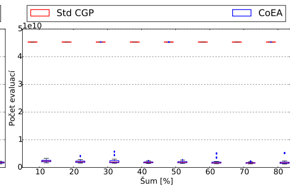
(f) Výstřelový 100 000 generací.
