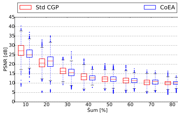
(a) Sůl a pepř 10 000 generací.
