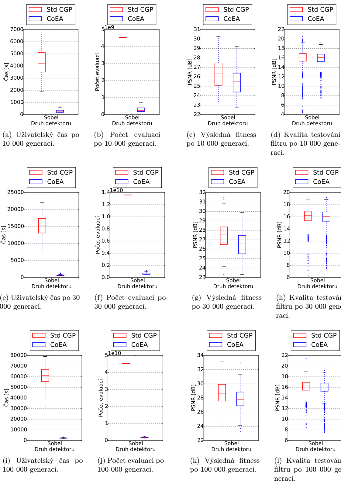
Obrázek C.25: Srovnání doby trvání, počtu evaluací, fitness konečného řešení a kvality přes testovací obrázky v úloze detektoru hran.
