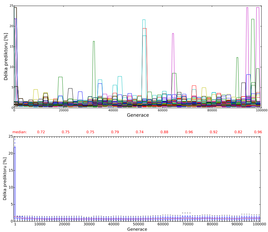
Obrázek C.4: Délka prediktorů v jednotlivých bězích - šum sůl a pepř intenzity 40%.
