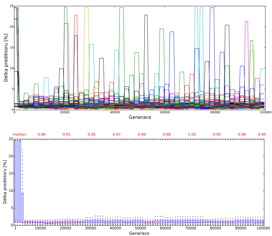
Obrázek C.12: Délka prediktorů v jednotlivých bězích - výstřelový šum intenzity 20 %.
