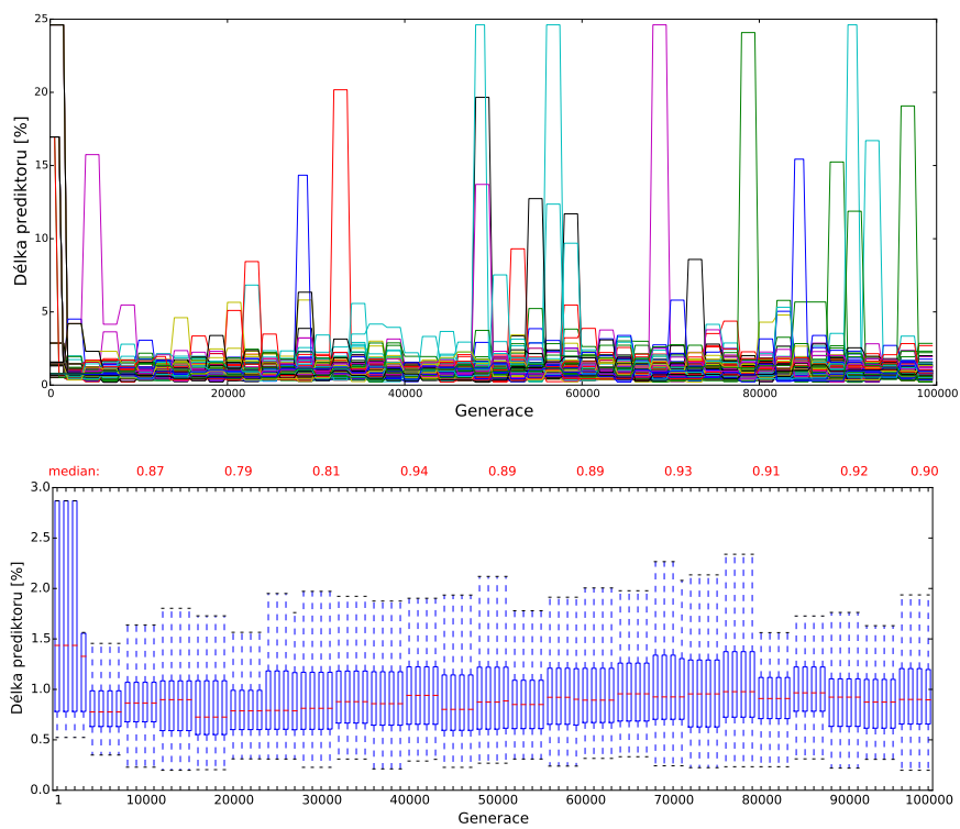
Obrázek C.13: Délka prediktorů v jednotlivých bězích - výstřelový šum intenzity 30 %.
