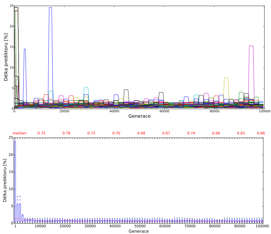
Obrázek C.16: Délka prediktorů v jednotlivých bězích - výstřelový šum intenzity 60 %.
