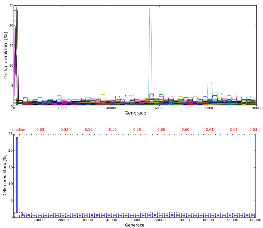
Obrázek C.17: Délka prediktorů v jednotlivých bězích - výstřelový šum intenzity 70 %.
