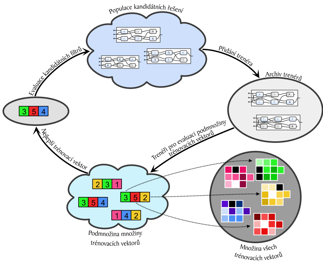
Obrázek 2.7: Koevoluce obrazových filtrů s trénovacími vektory.
