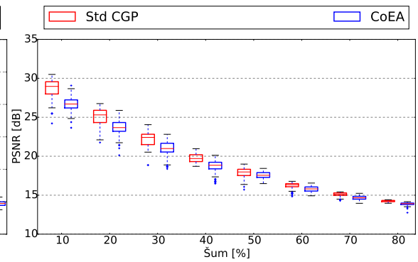
(b) Výstřelový 10 000 generací.
