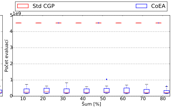
(b) Výstřelový 10 000 generací.
