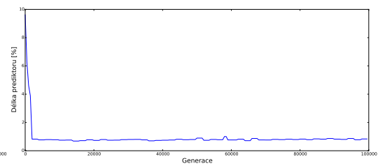
(b) Sůl a pepř 60%.
