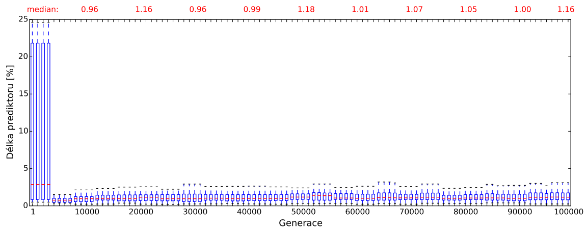
(a) 10% impulzní náhodný šum
