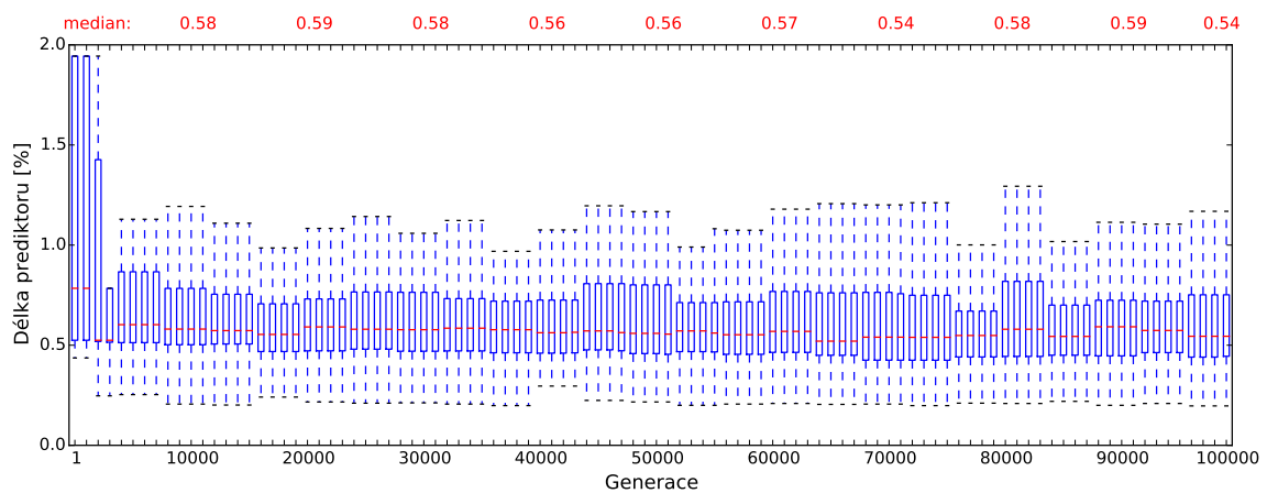
(c) 80% impulzní náhodný šum
