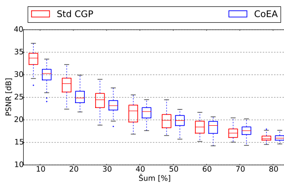
(e) Sůl a pepř 100 000.
