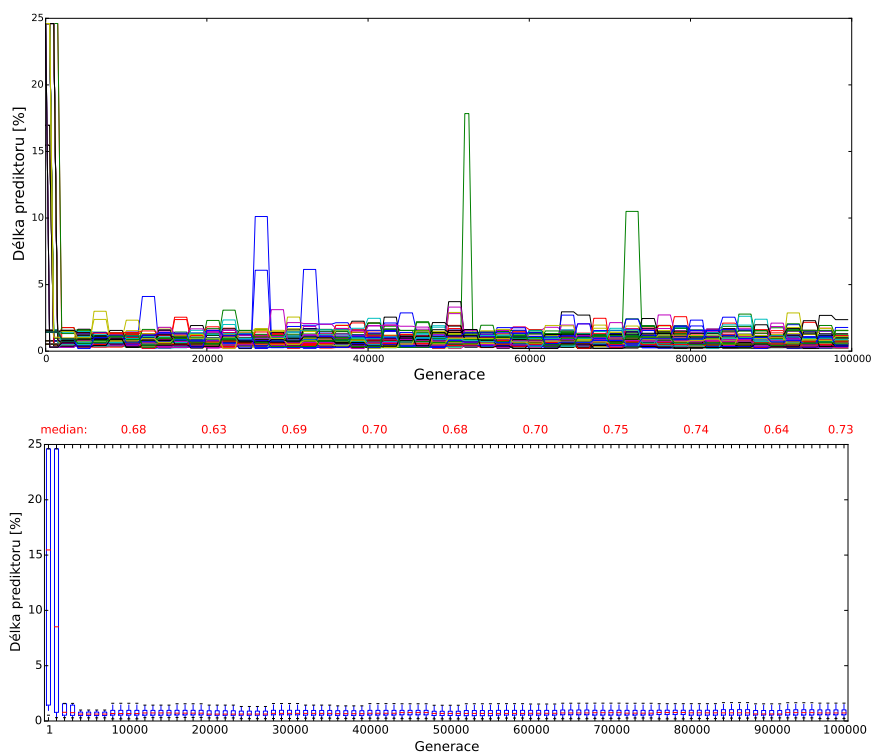
Obrázek C.7: Délka prediktorů v jednotlivých bězích - šum sůl a pepř intenzity 70%.
