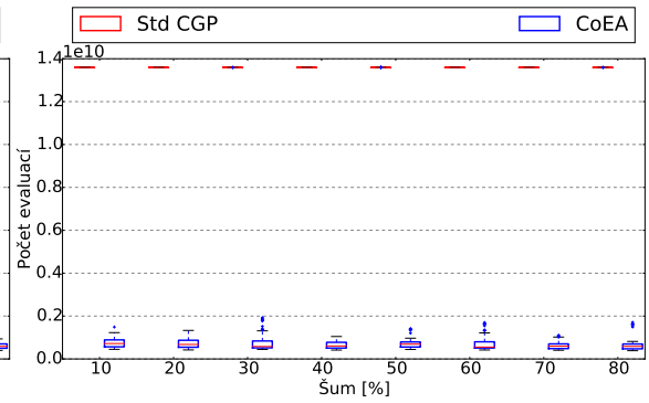
(d) Výstřelový 30 000 generací.
