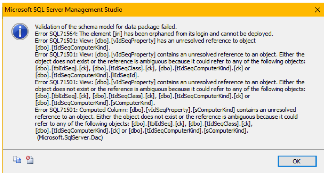
Obr. 9 Výsledek kontroly připravenosti databáze k přesunu do Microsoft Azure. (12)
