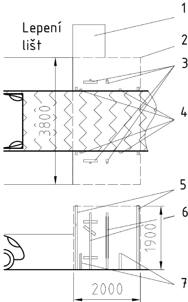
Obrázek 5-18 prostor měření boků vozidla
