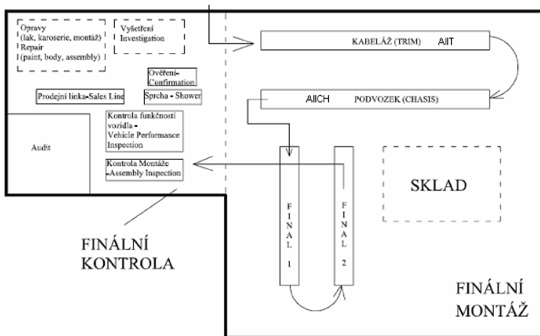
Obrázek 2-2 Rozvržení montážní linky a výstupní kontroly
