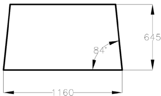
Obr. 5-8 – schematický návrh tvaru rámu
