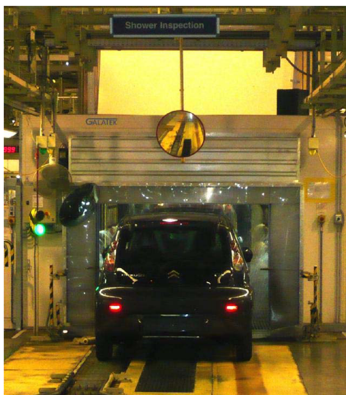
Obrázek 2-7 sprchový box
