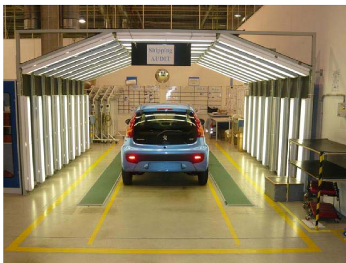
Obrázek 2-8 pracoviště auditu
