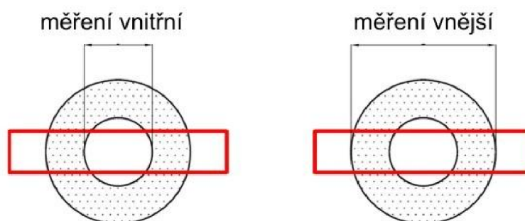
Obrázek 3-4 měření rozměrů
