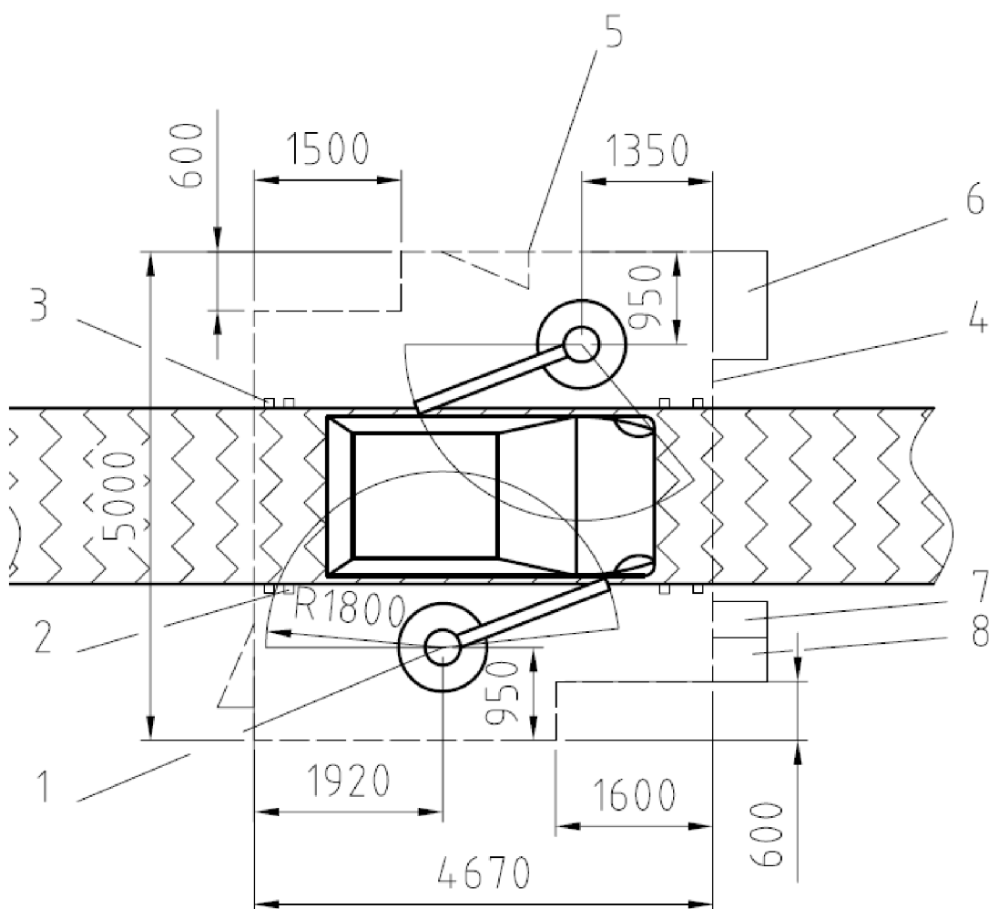
Obrázek 5-21 rozvržení robotizované pracoviště měření
