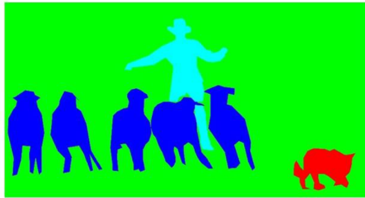
Sémantická segmentace
