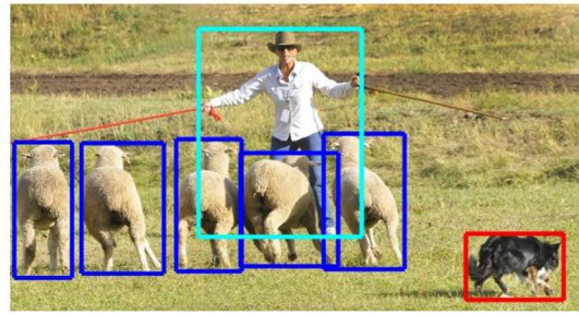
Detekce objektů
