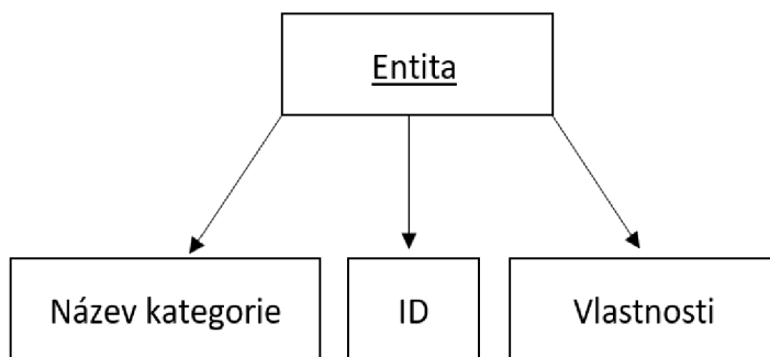
Obrázek 5: Schéma entity
