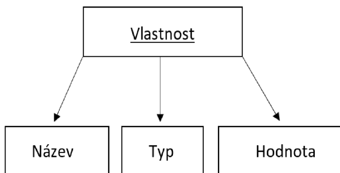
Obrázek 6: Schéma vlastnosti
