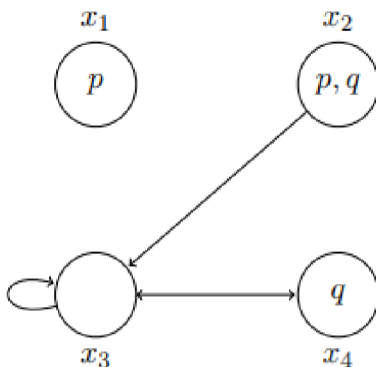
Obrázek 3: Kripkeho model s proposicemi p a q
