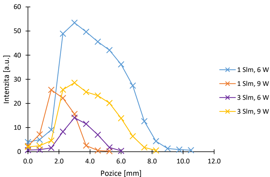
Obrázek 26: Graf průběhu integrální intenzity atomárního kyslíku (první spektrální čáry rozlišeného tripletu při 777,19 nm) v závislosti na vzdálenosti od konce aplikátoru
