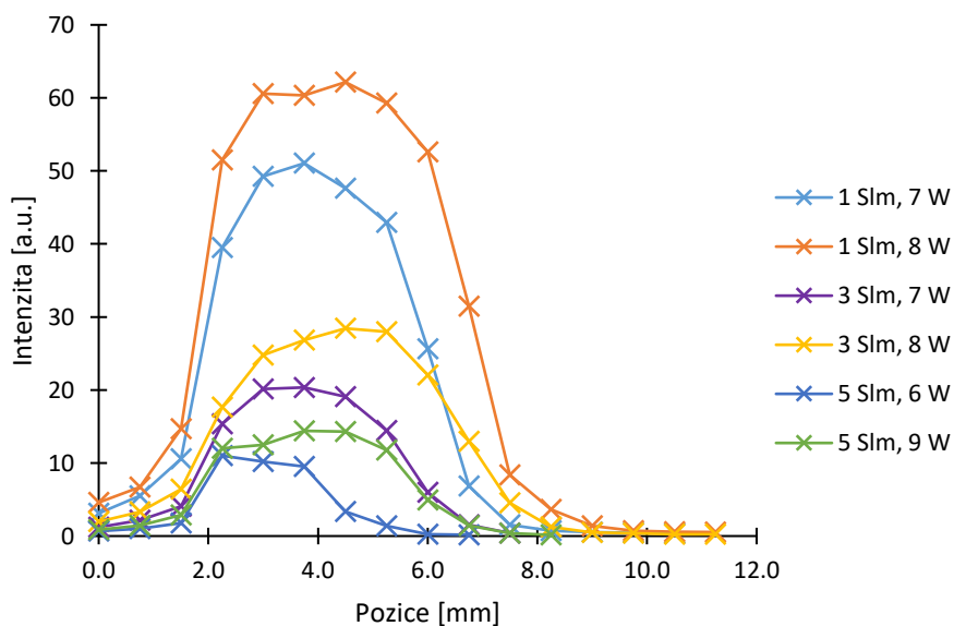
Obrázek 17: Graf průběhu integrální intenzity atomárního kyslíku (první spektrální čáry rozlišeného tripletu při 777,19 nm) v závislosti na vzdálenosti od konce aplikátoru
