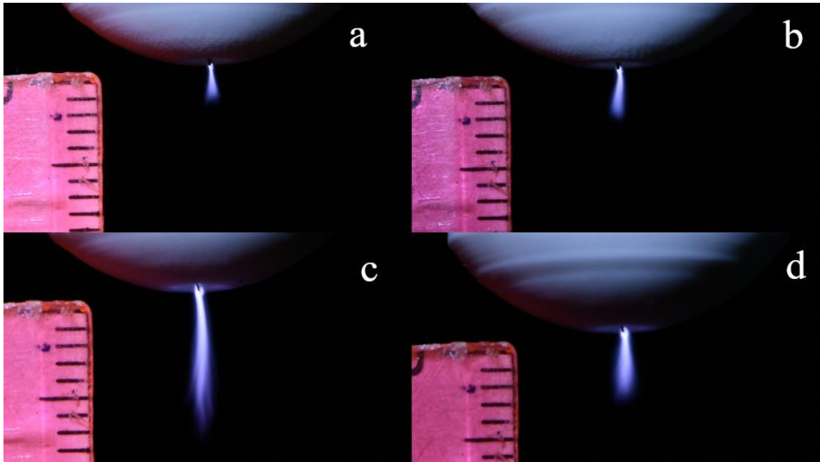
Obrázek 34: Fotografie výbojů aplikátoru s úhlem 30^\circ ; a – 1 Slm, 6 W; b – 3 Slm, 6 W; c – 1,6 Slm, 10 W; d – 3,5 Slm, 10 W
