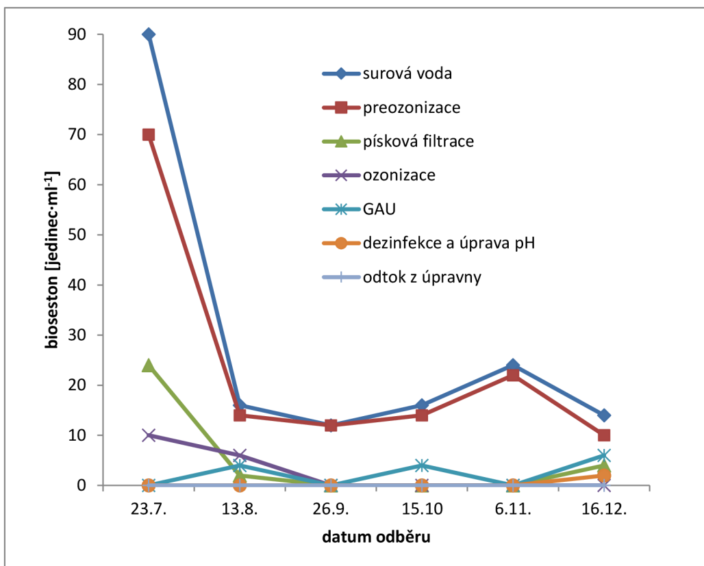
Obrázek 20: Bioseston vyjádřený v jedincích v surové vodě, v průběhu procesů technologie úpravy vody a na odtoku z ÚV Švařec
