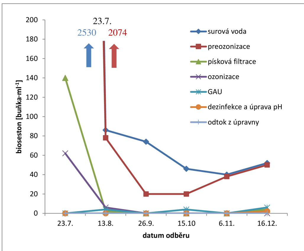
Obrázek 21: Bioseston vyjádřený v buňkách v surové vodě, v průběhu procesů technologie úpravy vody a na odtoku z ÚV Švařec
