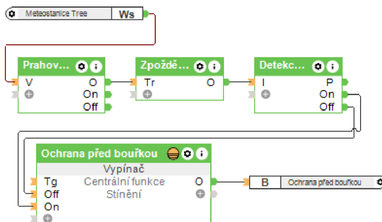
Obr. 18: Konfigurace funkce Ochrana před bouřkou
