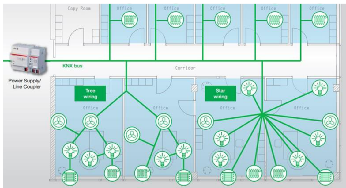
Obr. 4: Schéma popsaných topologií sítě [14]
