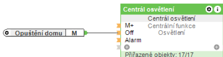
Obr. 15: Funkční blok Centrál osvětlení (vlastní zdroje)
