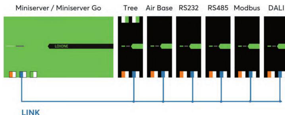
Obr. 9: Schéma zapojení Extensionů a Miniserveru [10]
