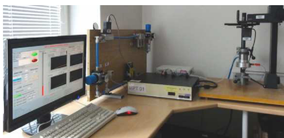
Obrázek 11 - Zařízení MPT 01 [56]
