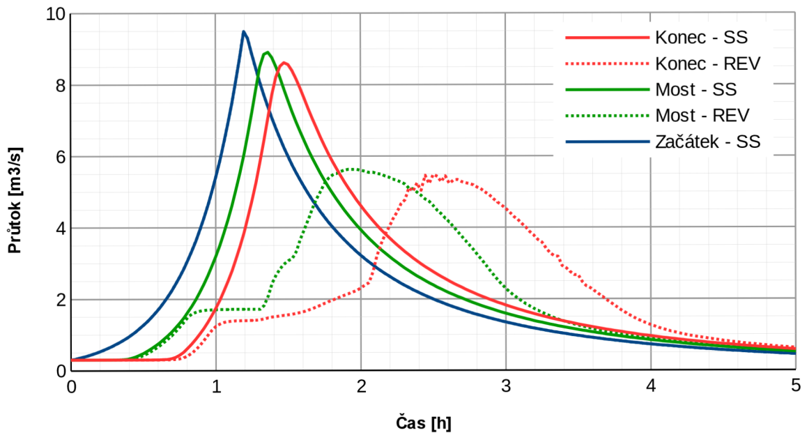
Obr. 3.19: Varianta A1 - Graf transformace povodňové vlny Q 5
