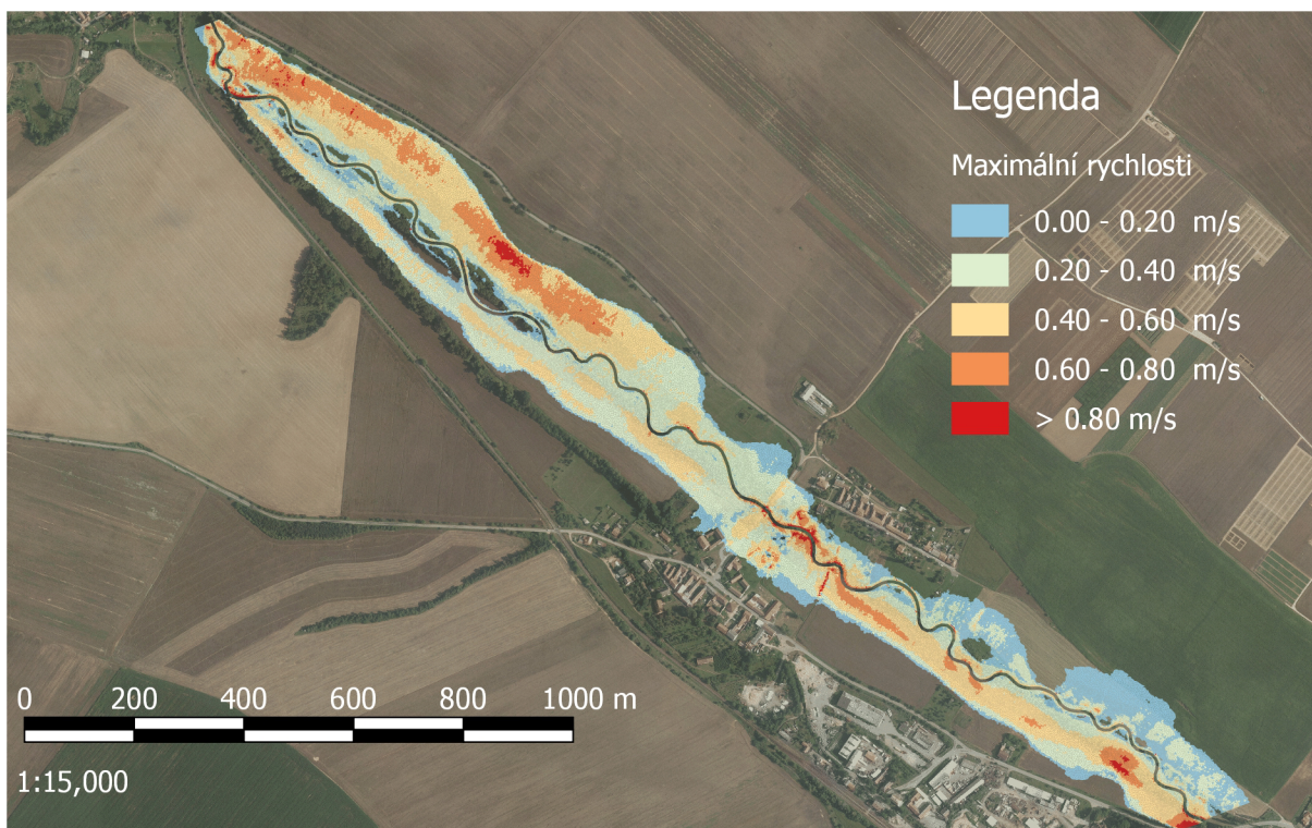
Obr. 4.7: Zobrazení maximálních rychlostí v nivě při hydrogramu 2x Q_1 , Q_{100} varianty B4
