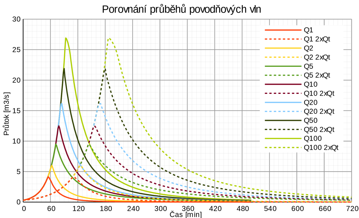
Obr. 3.6: Graf porovnání průběhů povodňových vln Q_t a 2x Q_t
