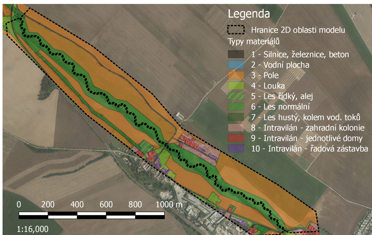
Obr. 3.12: Mapa drsností v revitalizované variantě A1
