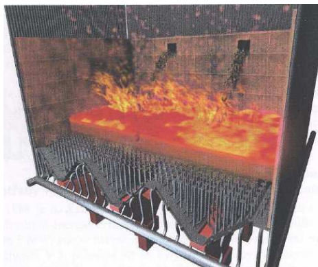
Obr. 2.5 Kotel se spalováním ve fluidní stacionární vrstvě [2]
