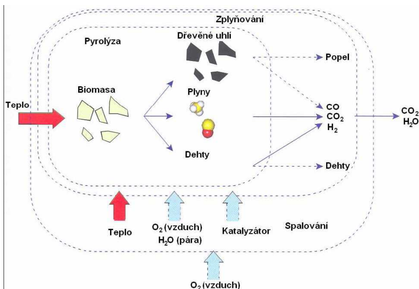
Obr. 2.6 Schéma zplyňování [2]
