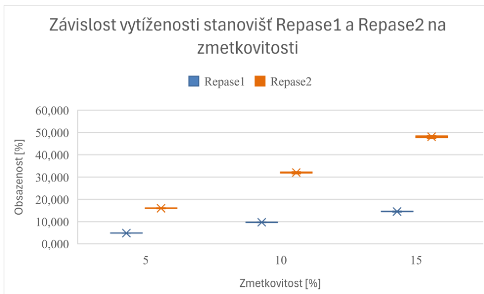
Obr. 17 Závislost vytiženosti stanovišť Repase1 a Repase2 na zmetkovitosti
