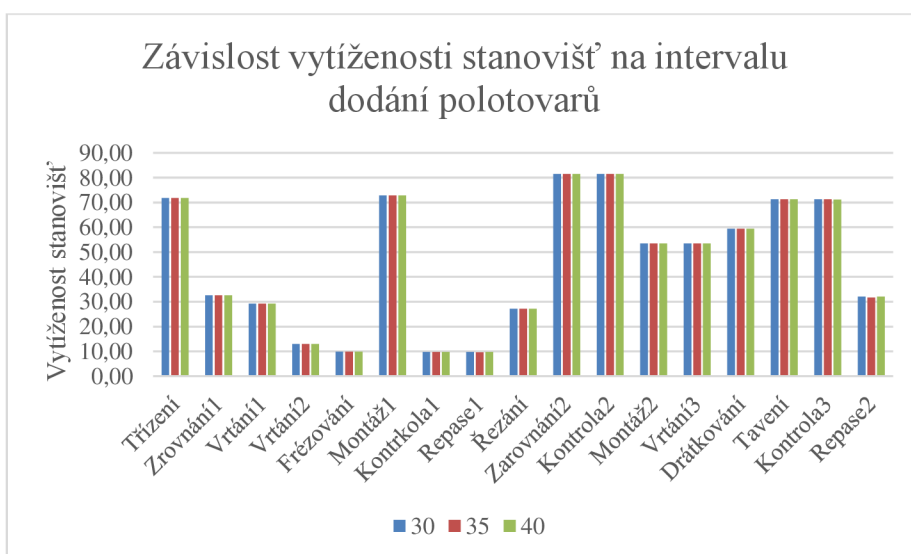
Obr. 19 Závislost vytiženosti stanovišť na intervalu dodání polotovaru
