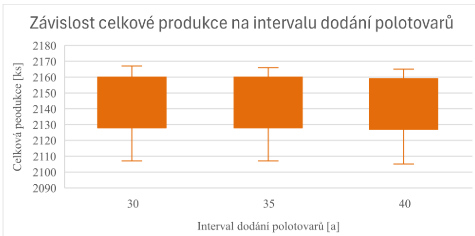
Obr. 18 Závislost celkové produkce na intervalu dodání polotovaru
