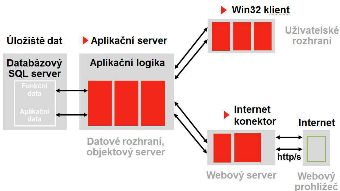
Obrázek 2: Architektura QI
