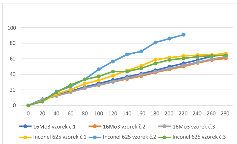
Obr. 59 Porovnání hodnot Inconel 625 a 16Mo3 při 975°C.
