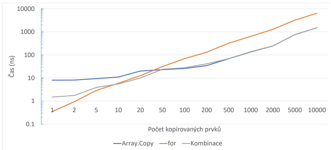
Obrázek 4.1: Délka kopírování různých algoritmů v závislosti na počtu prvků
