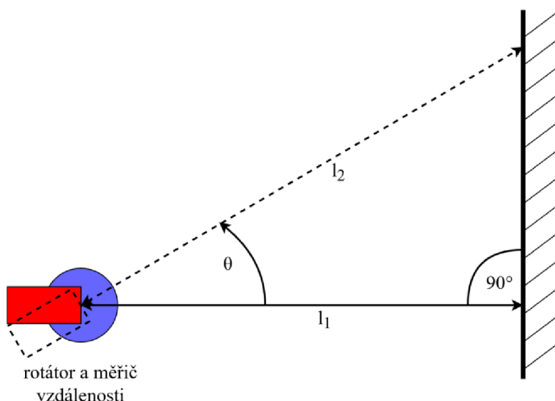
Obrázek 7.7 Experiment pro zjištění opakovatelnosti nastavení úhlu rotátorem Edelkrone, pohled shora
