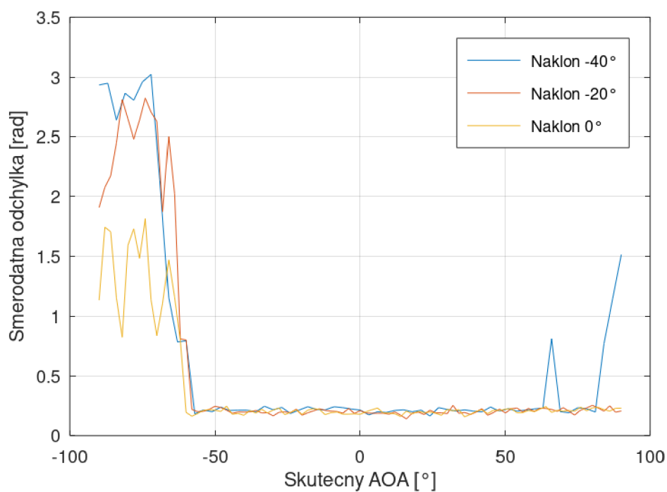
Obrázek 7.5 Průběh směrodatné odchylky pro různé úhly náklonu
