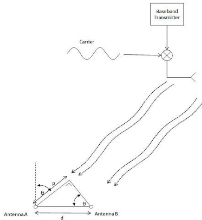
Obrázek 5.6 Princip PDOA [20]
