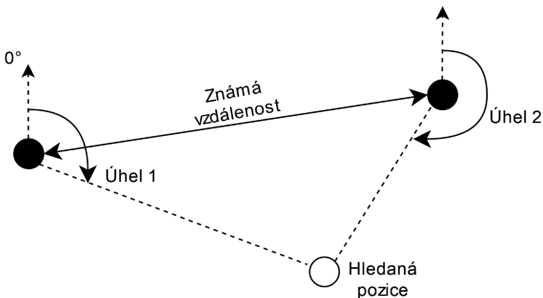
Obrázek 5.5 Příklad triangulace
