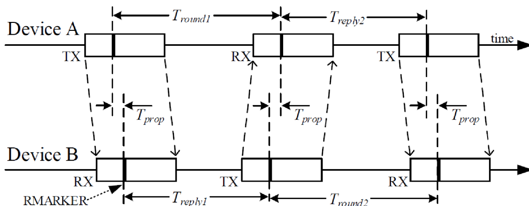
Obrázek 5.2 Dvoustranné TWR s použitím 3 zpráv [16]
