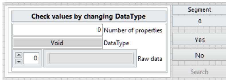
Obr. 7.6: Uživatelské prostredie pre kontrolu správnosti Raw dát s výberom dátového typu v prostredí LabVIEW.
