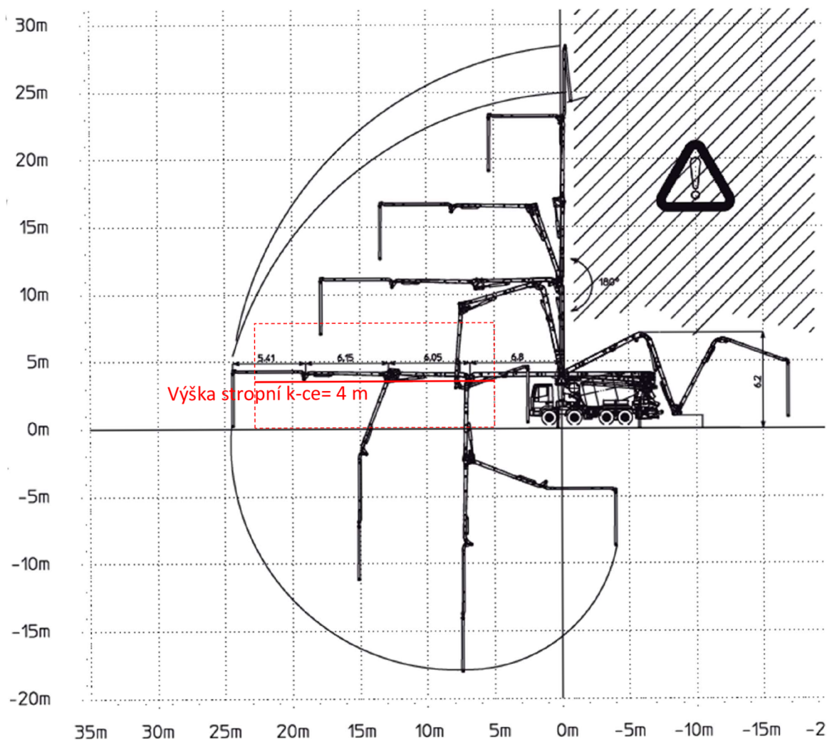
Obr. č. 28 – Diagram dosahu výložníku čerpadla domíchávače
