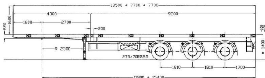
Obr. č. 22 – Návěs Faymonwille - rozměry
