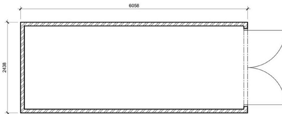
Obr. č. 18 – Půdorys skladového kontejneru
