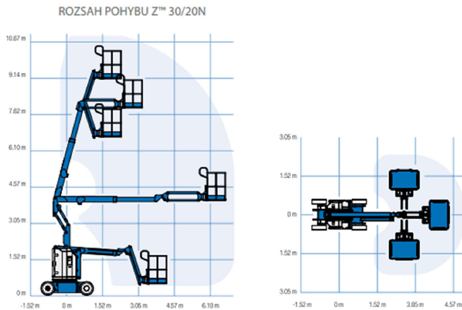
Obr. č. 30 – Montážní plošina – rozsah pohybu
