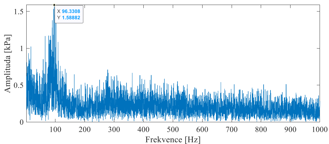
Obr. 8.9 – FFT, \sigma = 0,163
