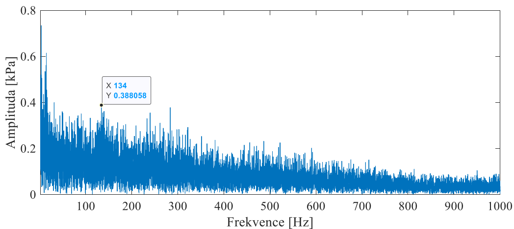
Obr. 8.5 – FFT, \sigma = 0,244
