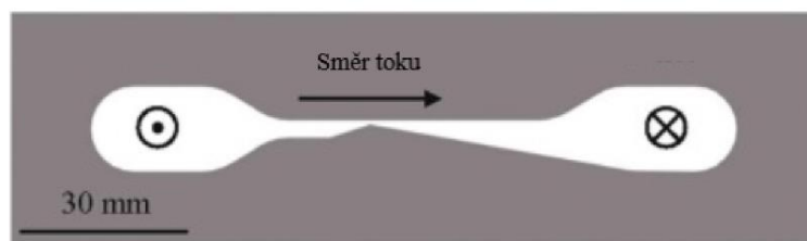
Obr. 3.2 – Geometrie dýzy [24]
