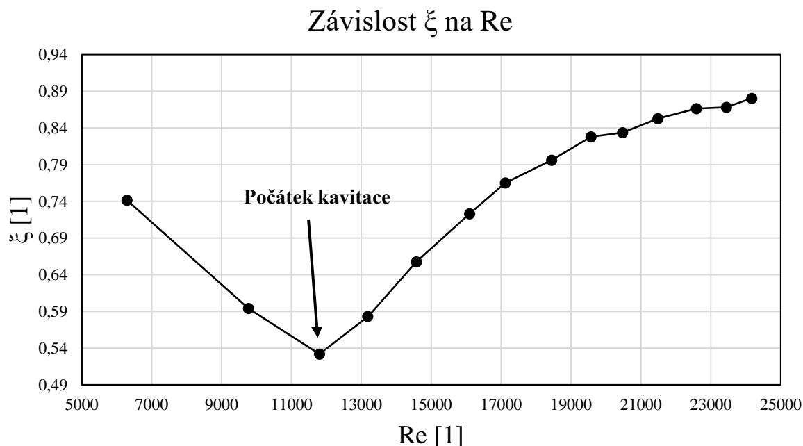
Obr. 4.9 – Závislost ztrátového součinitele na Reynoldsově čísle
