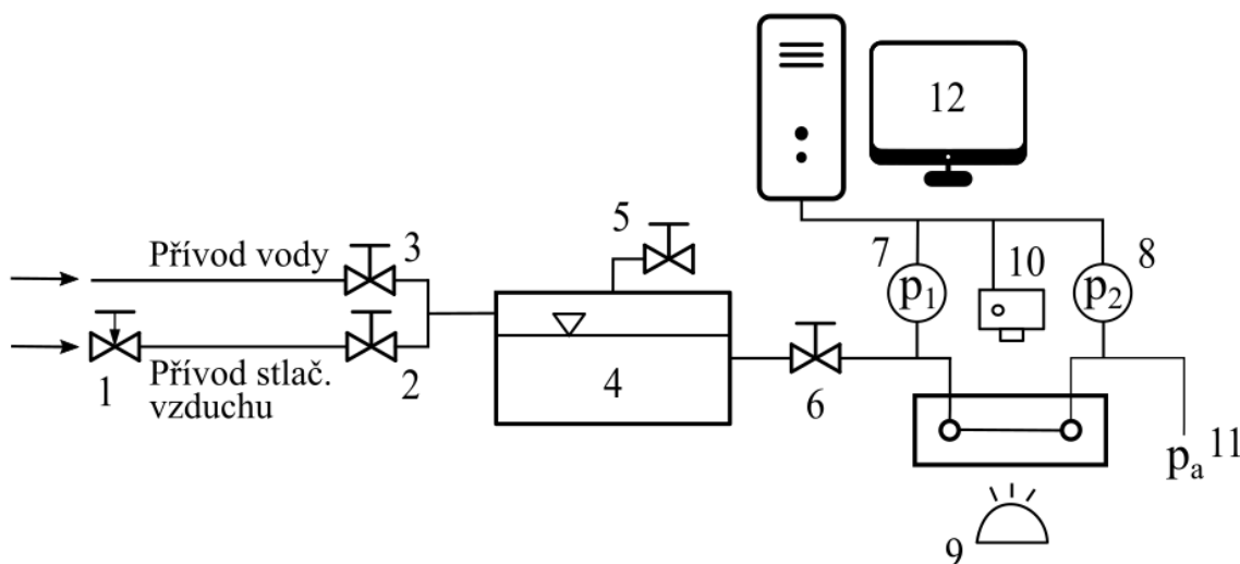
Obr. 4.1 – Schéma měřicí tratě
