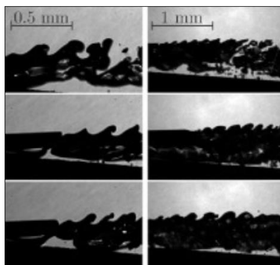
Obr. 2.11 – Kolaps kavitační bubliny [24]
