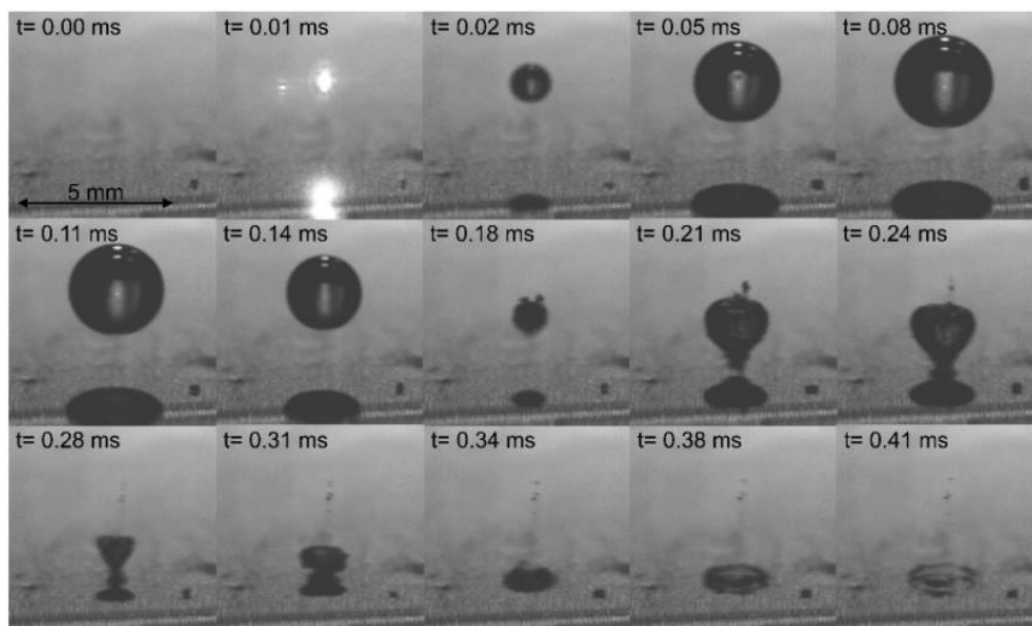
Obr. 2.10 – Kolaps kavitační bubliny v blízkosti stěny [23]
