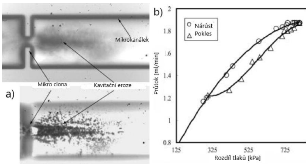
Obr. 2.7 – a) kavitační eroze, b) hystereze [17][18]
