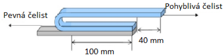
Obrázek 1: schéma peel testu [10].
