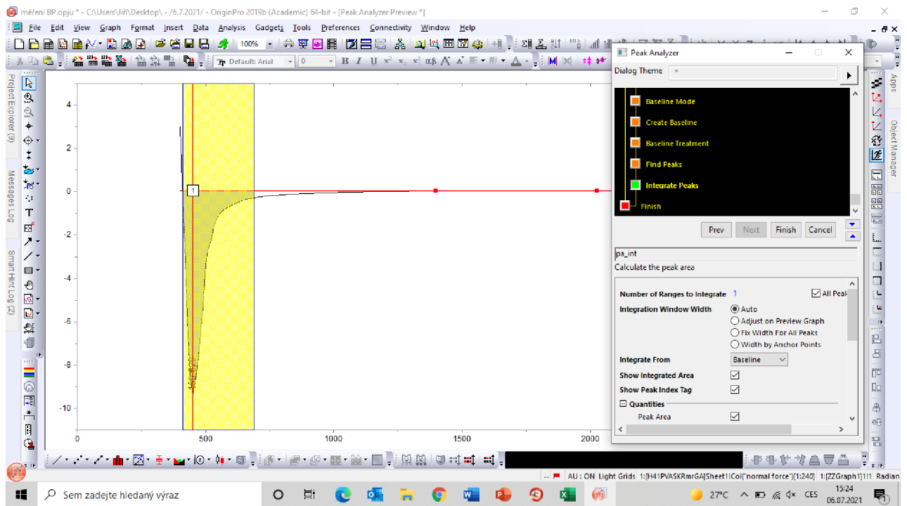
Obrázek 17: Vyhodnocení dat v programu Origin s ohraničenou plochou adhezni práce.
