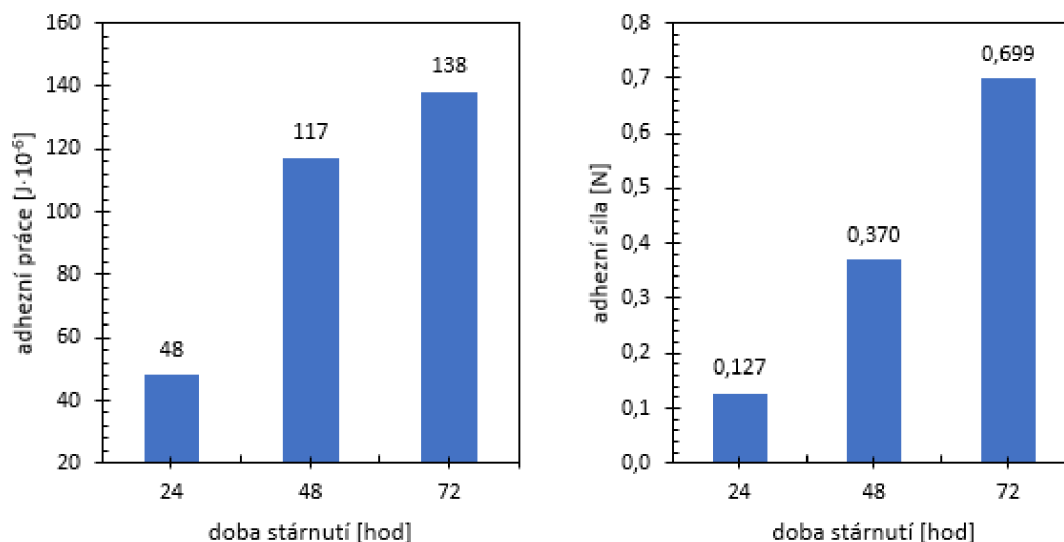
Obrázek 30: Na levé straně závislost adhezní práce na době stáří. Na pravé straně závislost adhezní síly na době stáří (PVA s přidavkem 2 ml GA a 30 minutami mražení).
