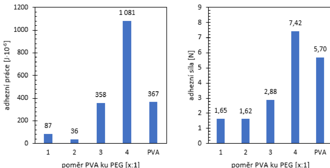
Obrázek 34: Na levé straně závislost adhezní práce na poměru PVA ku PEG. Na pravé straně závislost adhezní síly na poměru PVA ku PEG. (Hydrogely s přidavkem GA).
