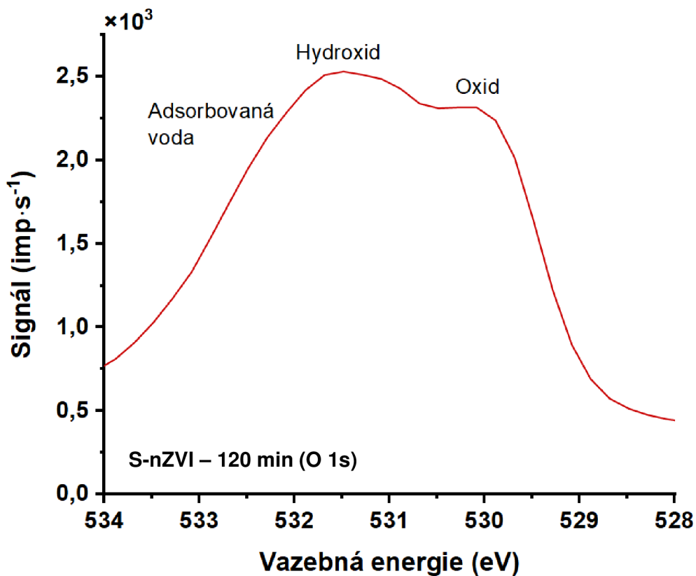
Obr. 23: XPS spektrum s vysokým rozlíšením v oblasti O 1s vzorku častíc S-nZVI po 120 min v čisté DO/DI vodě.
