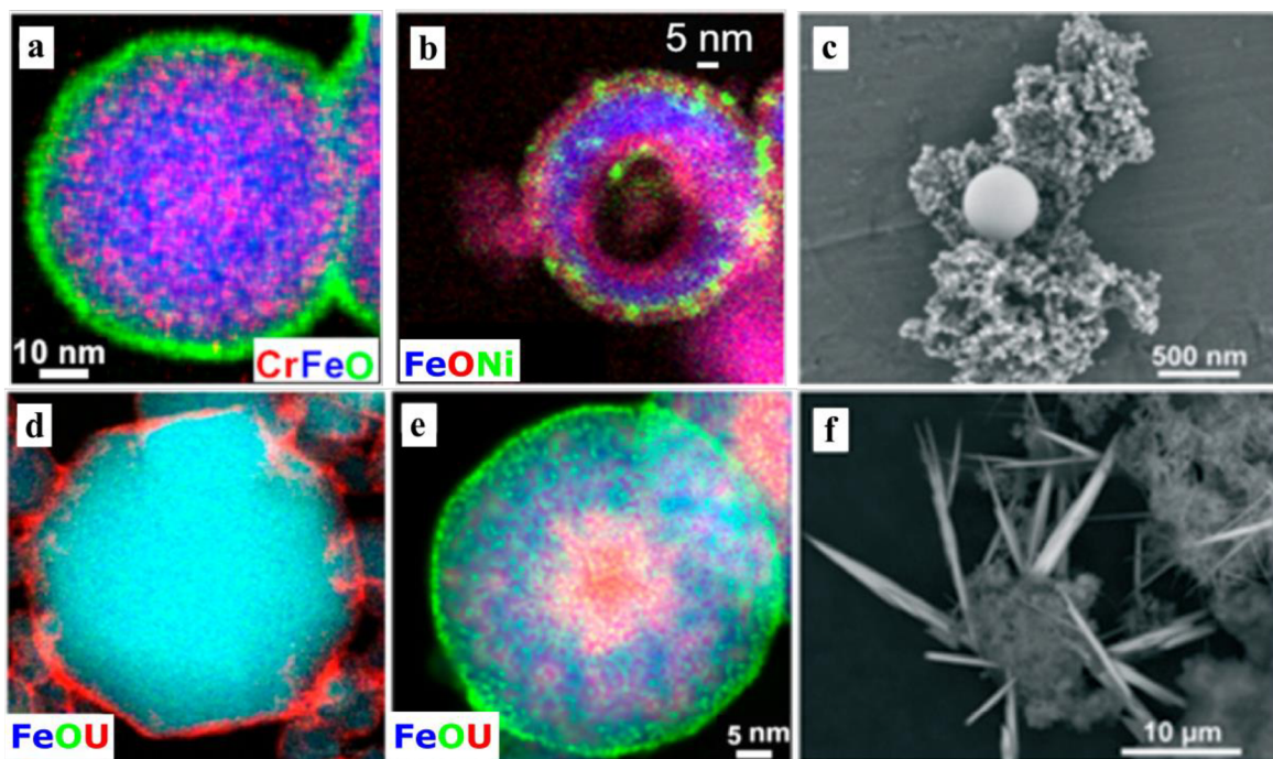
Obr. 12: Vzhled částic nZVI po reakci s těžkými kovy. Prvkové mapování pomocí STEM-EDS: a) reakce s K_2Cr_2O_7 , b) reakce s NiCl_2 , d) částice hematitu ( \alpha-Fe_2O_3 ) a e) nZVI po reakci s \cdot UO_2(NO_3)_2 . Snímky d, e jsou ve stejném měřítku. c, f) snímky částic po reakci s Na_2SeO_3 pořízené pomocí SEM. Doba reakce byla ve všech případech 24 h. Převzato z [68] (snímek a), [164] (b), [163] (c,f) a [165] (d,e).
