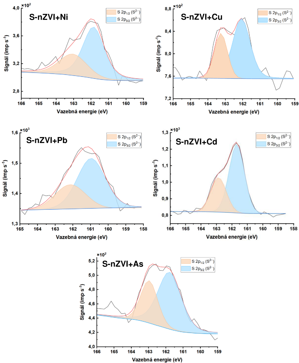
Obr. P.3: Proložená XPS spektra v oblasti síry (S 2p) vzorků částic S-nZVI po 120 min reakce s těžkými kovy.
