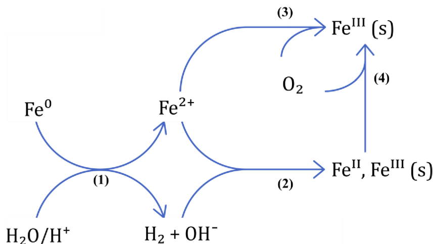
Obr. 5: Schéma reakcí nanočástic železa ve vodném prostředí. Povrch částic koroduje – elementární železo se oxiduje při reakci s vodou (1) za vzniku hydroxidových iontů a vodíku, následují srážecí reakce (2) a (3). Mezi vzniklými oxidy, hydroxidy a hydroxid-oxidy železa v oxidačních stavech II nebo III dochází k transformacím (4). Podle [58].
