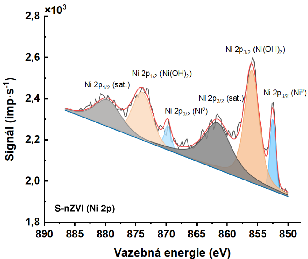
Obr. 26: Proložené XPS spektrum v oblasti Ni 2p vzorku částic S-nZVI po 120 min reakce.
