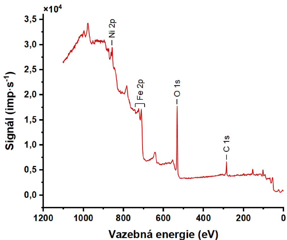
Obr. P.4: Přehledové spektrum vzorku částic nZVI po 120 min reakce s Ni(II).
