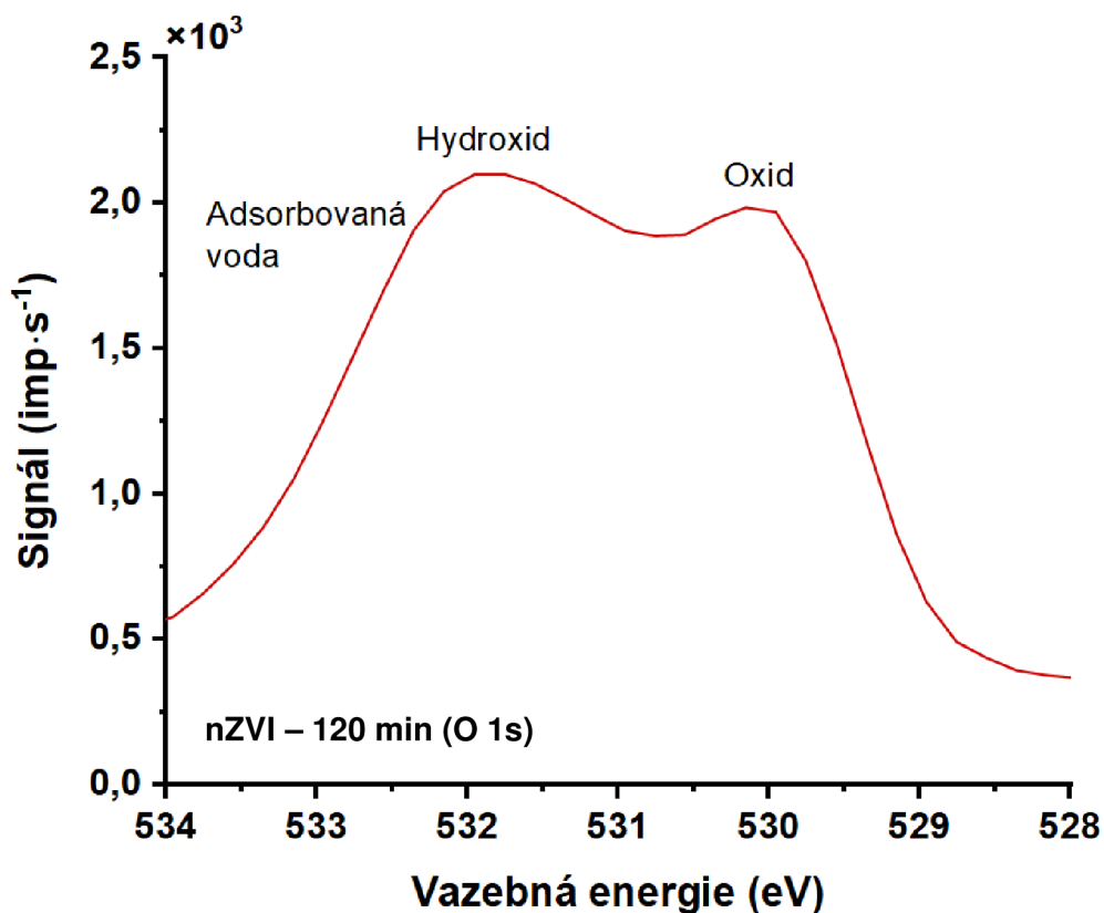
Obr. 22: XPS spektrum s vysokým rozlíšením v oblasti O 1s vzorku častíc nZVI po 120 min v čisté DO/DI vodě.
