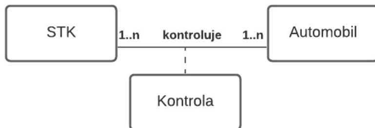
Obrázok 9: OOP – typy vzťahov – príklad asociačnej triedy – vyjadrenie pomocou UML
