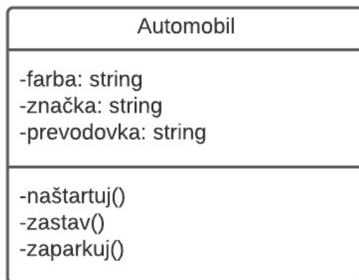
Obrázok 5: OOP – príklad triedy – vyjadrenie pomocou UML
