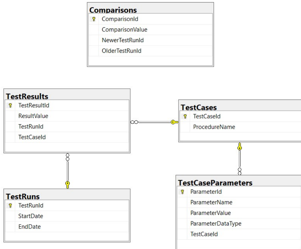
Obrázok 32: Návrh databázy nástroja
