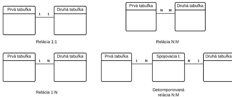
Obrázok 13: Kardinalita vzťahov medzi tabuľkami v entitno-relačnom modeli
