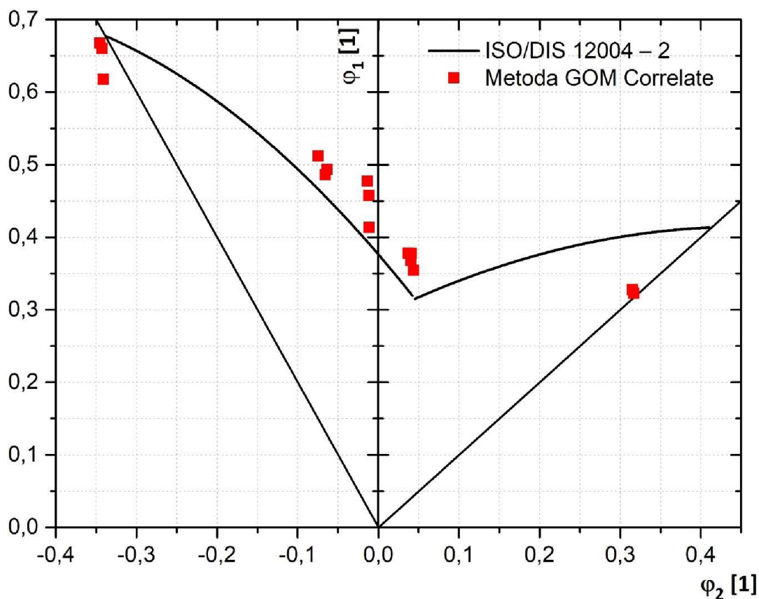
Obr. 45 Diagram mezních přetvoření získaný metodou GOM Correlate
