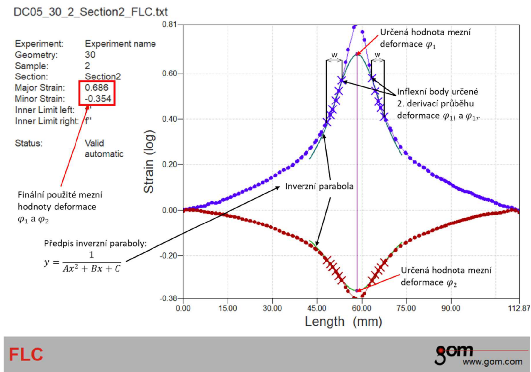
Obr. 37 Určení hodnot mezních deformací – vzorek 30_2
