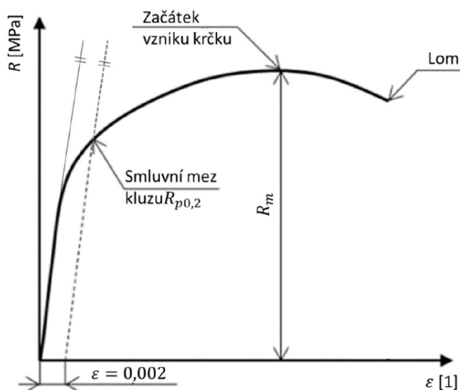
Obr. 14 Smluvní diagram R - \epsilon [11]
