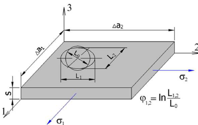
Obr. 15 Stabilita procesu tváření [16]
