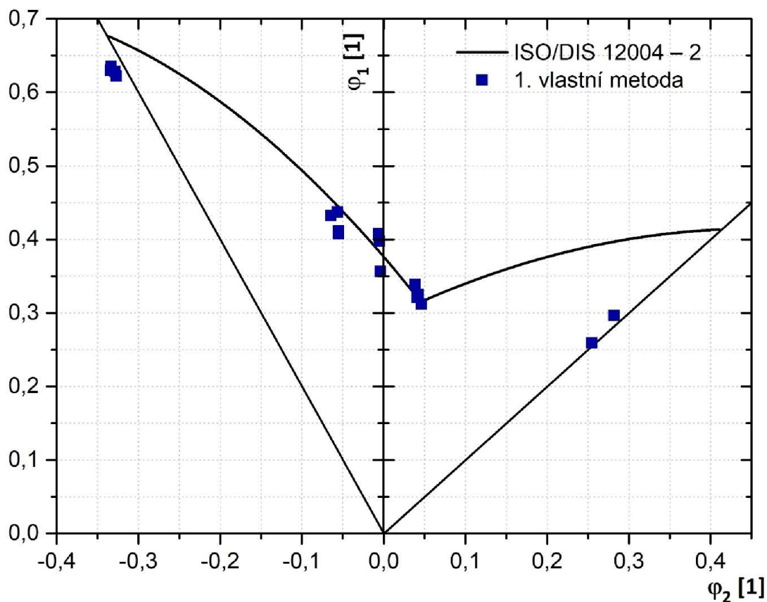
Obr. 46 Diagram mezních přetvoření získaný 1. vlastní metodou
