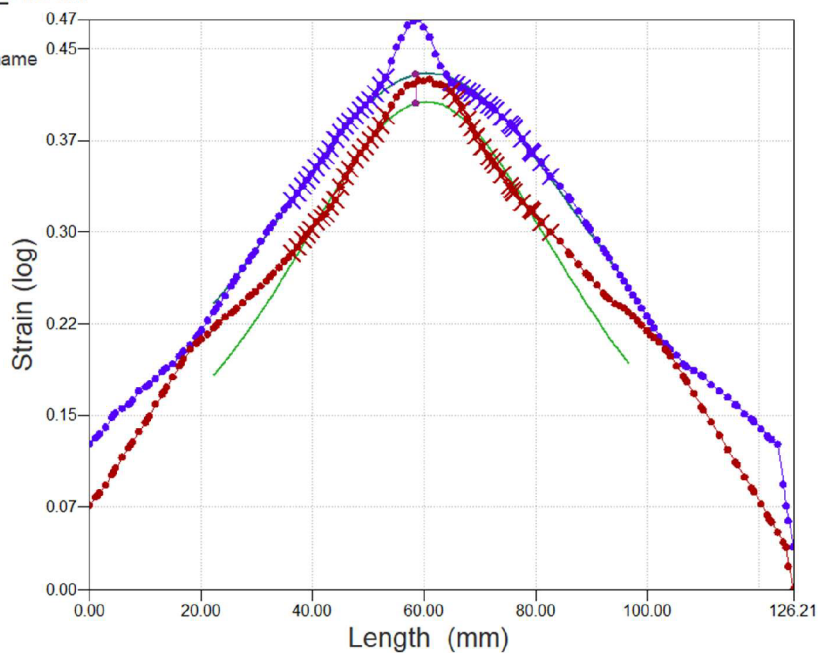
Obr. 39 Určení hodnot mezních deformací – vzorek HBT_2
