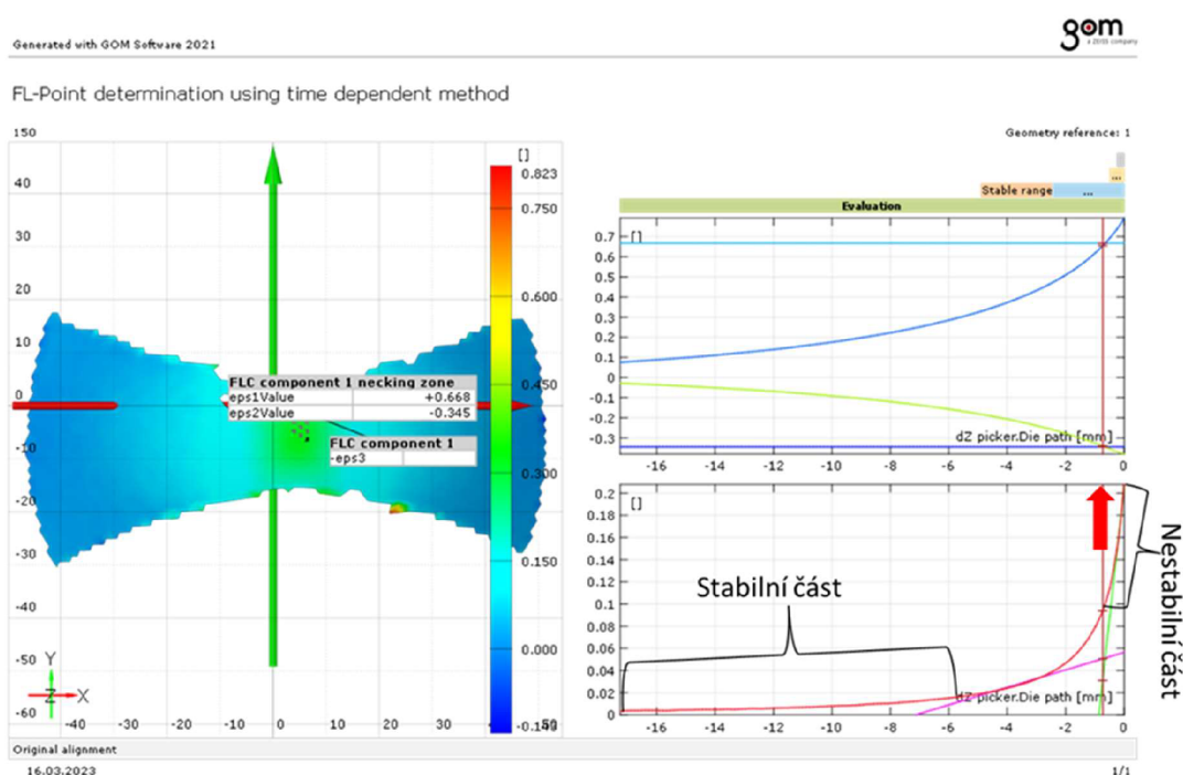
Obr. 40 Metoda založená na gradientu deformace – metoda GOM Correlate
