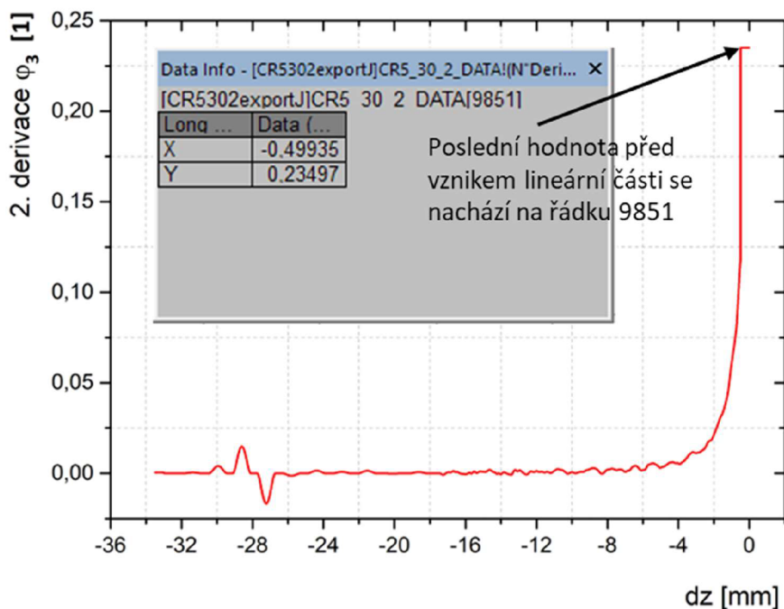
Obr. 41 Druhá derivace \varphi_3/dz
