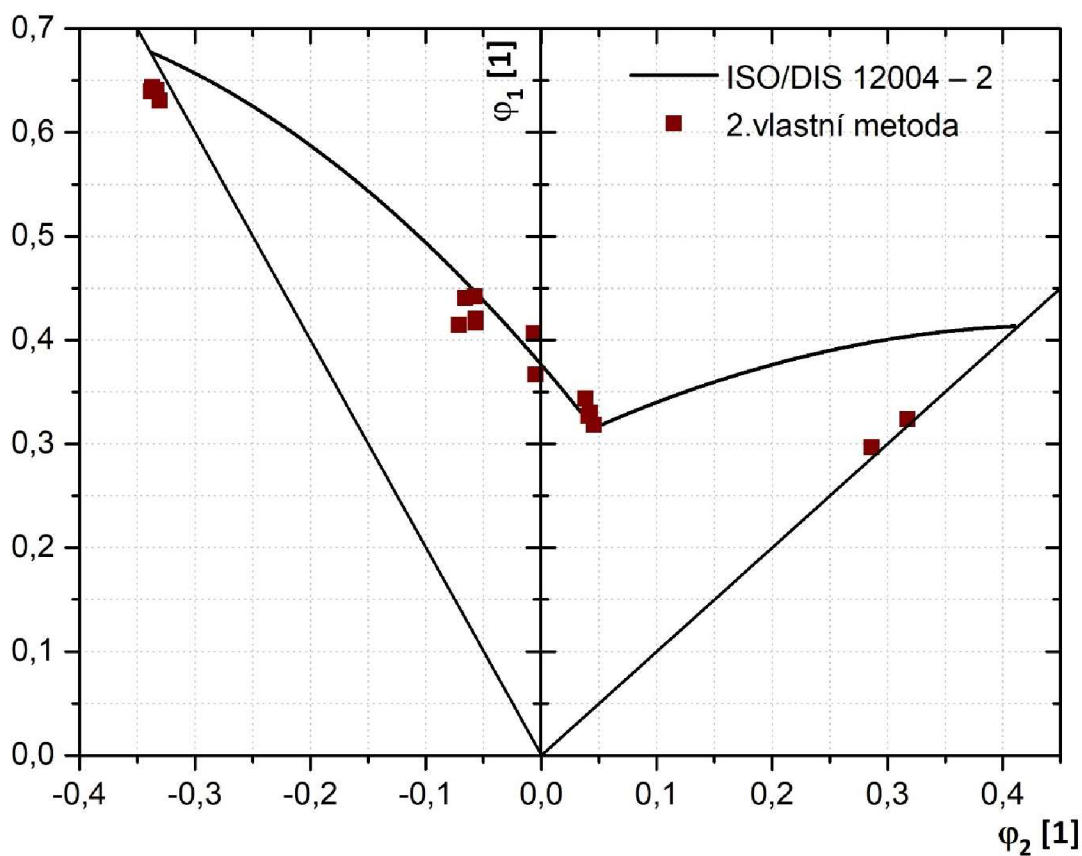
Obr. 47 Diagram mezních přetvoření získaný 2. vlastní metodou
