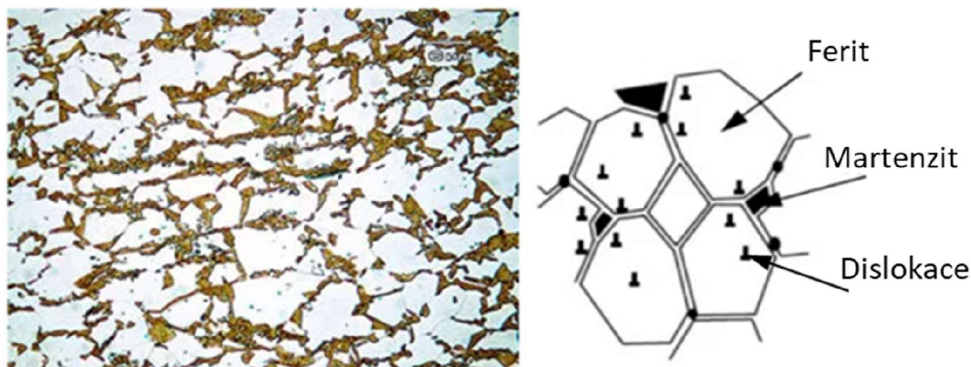
Obr. 8 Mikrostruktura DP oceli (vlevo) a schéma DP oceli (vpravo) [7]
