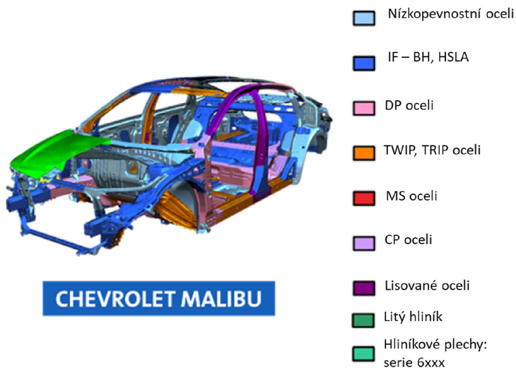
Obr. 3 Materiály karosérie automobilu Chevrolet Malibu [5]
