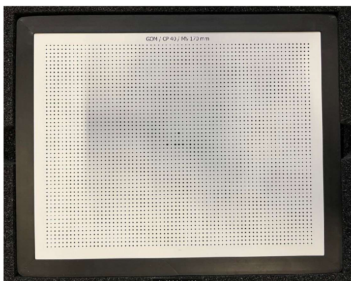
Obr. 32 Kalibrační destička GOM / CP40 / MV 170 mm
