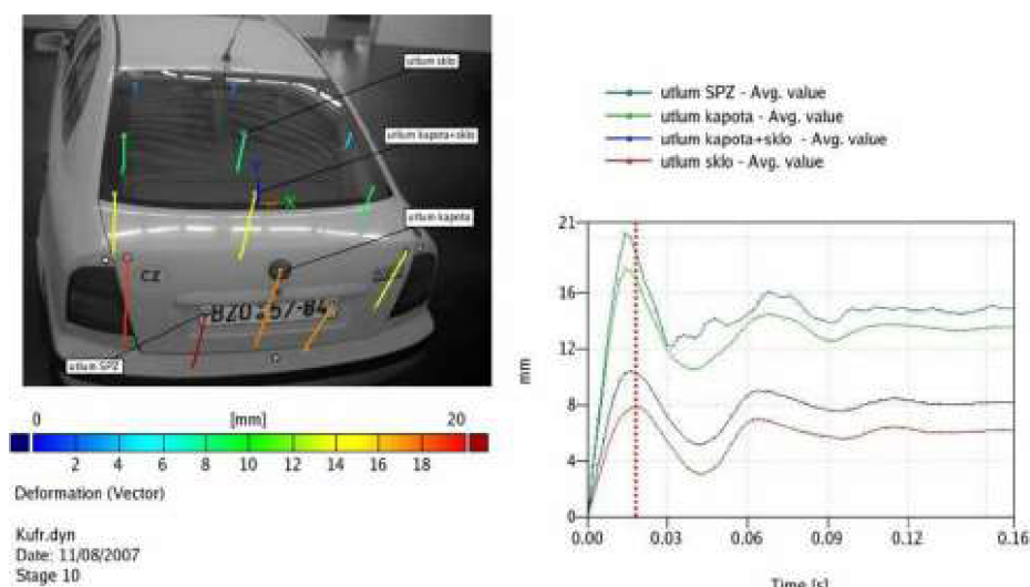
Obr. 22 Útlum pátých dveří Škoda Octavia [23]
