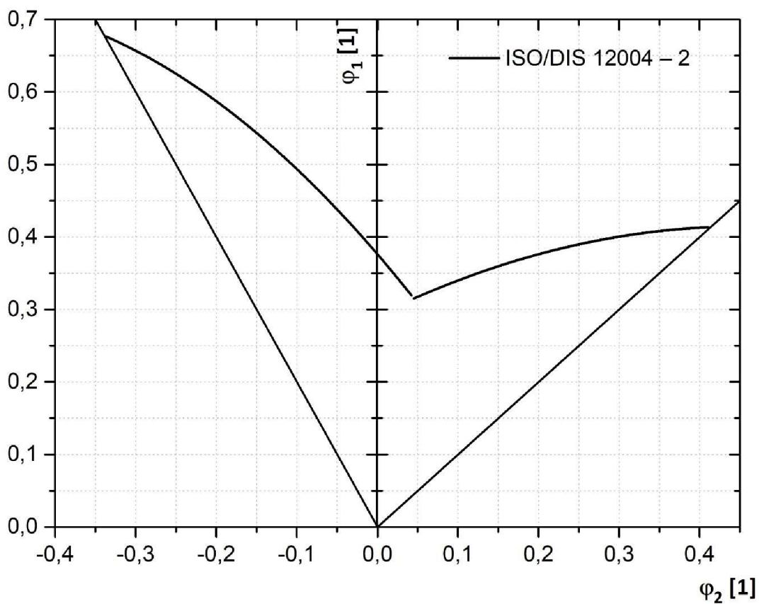
Obr. 44 Diagram mezních přetvoření získaný normovanou metodou ISO/DIS 12004 – 2
