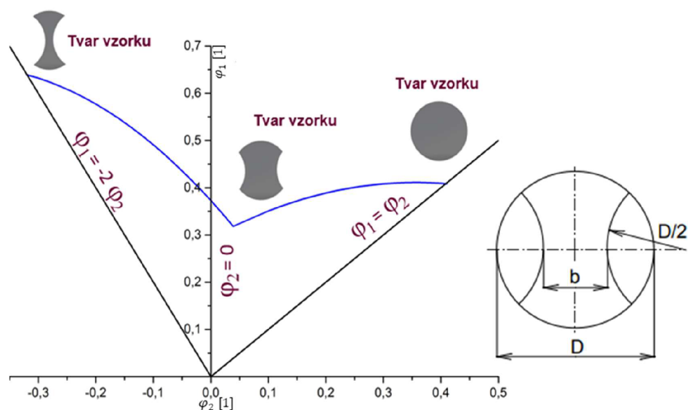
Obr. 18 Ukázka šířky vzorků pro jednotlivé části FLD (vlevo) [16] a tvar zkušebního tělesa (vpravo) [15]
