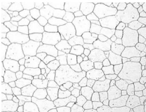
Obr. 5 Mikrostruktura oceli 180 BH [7]
