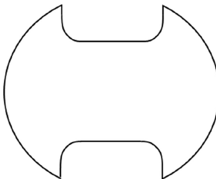
Obr. 17 Tvar zkušební tělesa pro Nakazima test
