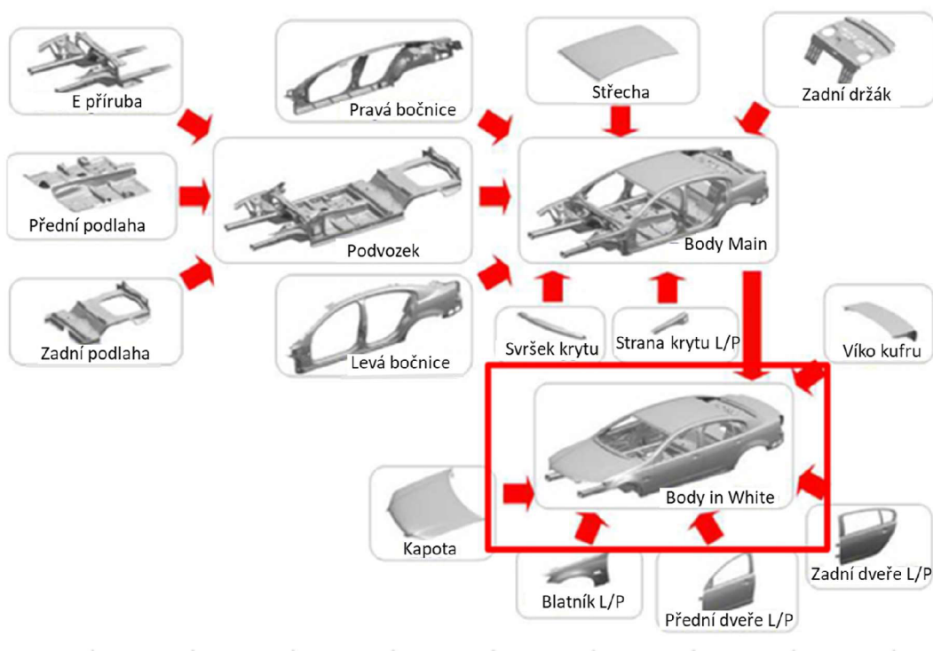
Obr. 2 Složení BiW [4]
