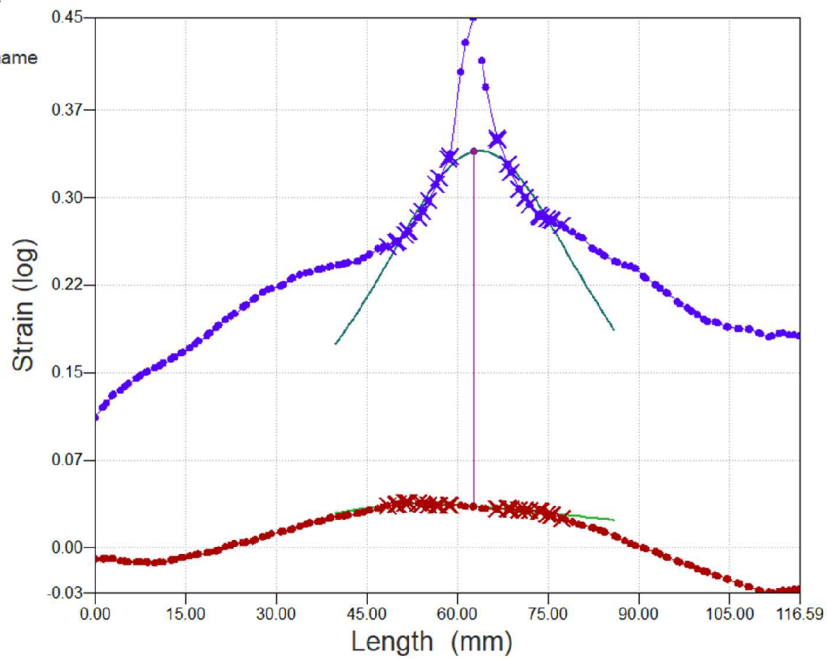
Obr. 38 Určení hodnot mezních deformací – vzorek 120_3
