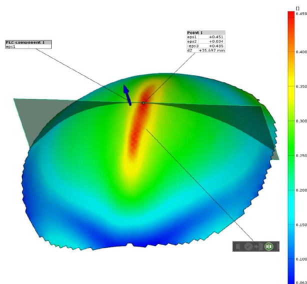
Obr. 25 Rozložení deformace \varphi_1 na vzorku
