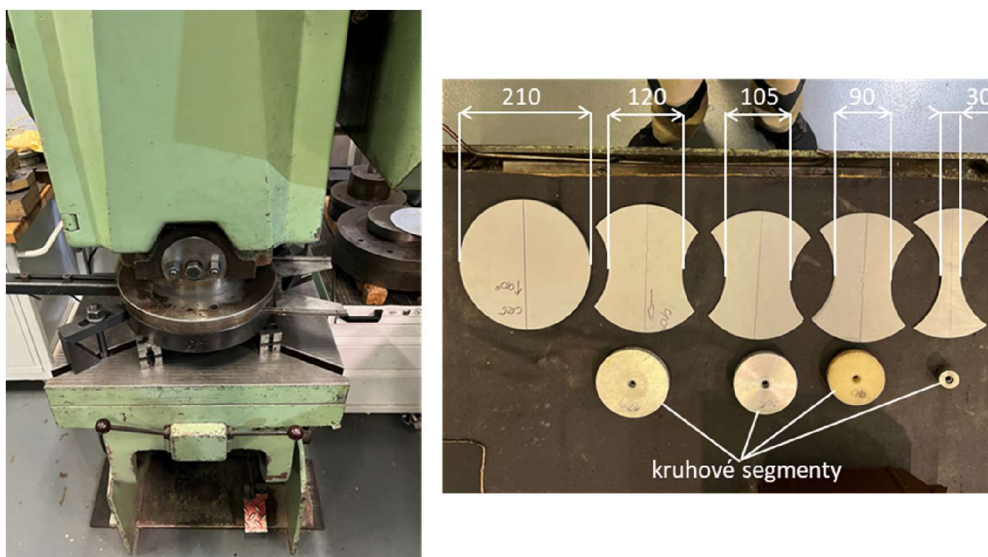
Obr. 29 Mechanický lis LEN – P 40 se střížným nástrojem (vlevo) a jednotlivé tvary vzorků s dorazy (vpravo)
