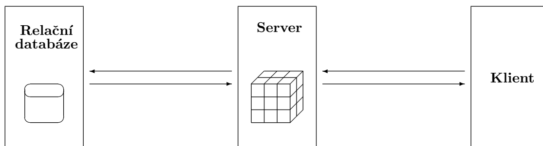
Obrázek 4.5: Schéma rozptření vrstev systému Hybrid OLAP
