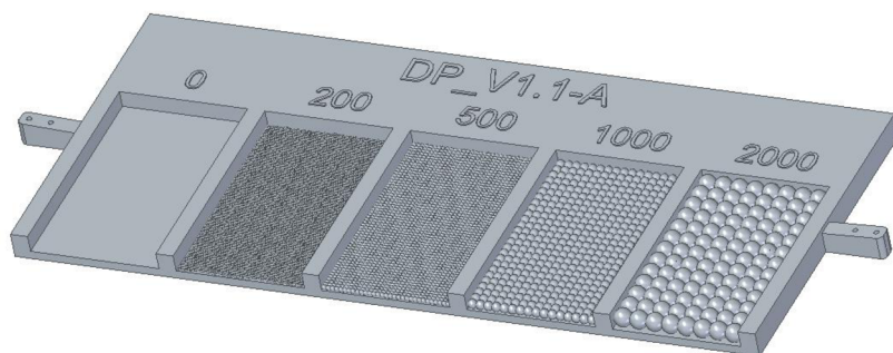
Obr. 20 CAD model vzorkovníku se vzory modifikovaných povrchů v prostředí softwaru SolidEdge 2020
