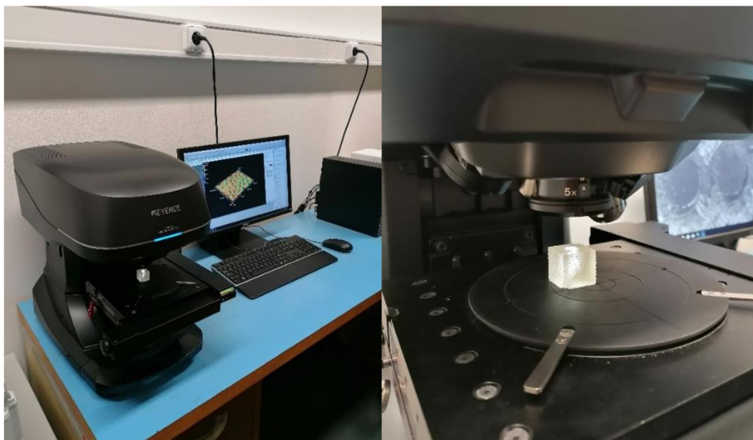
Obr. 35 Laserový skenovací mikroskop VK-X1000 (vlevo), detail měření střední aritmetické odchylky R_a na povrchu plně kostky (vpravo)
