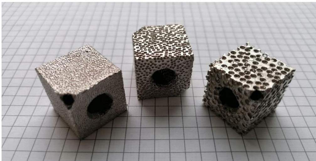
Obr. 47 Pokovené struktury polymer – kov E-d0,5-1(SLA), E-d1-1(SLA) a E-d2-1(SLA) zhotovené z odlehčených kostek
