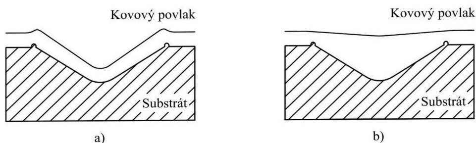
Obr. 12 Schematické znázornění vyrovnávacího účinku galvanických lázní [23] a) bez leskutvorných přísad, b) s přidávkem leskutvorných přísad
