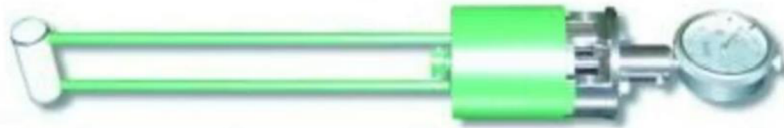
Obr. 17 IS – metr pro měření vnitřního pnutí v kovových povlácích [39]
