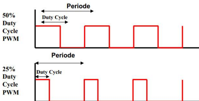
Obrázok 5.4 PWM[11]
