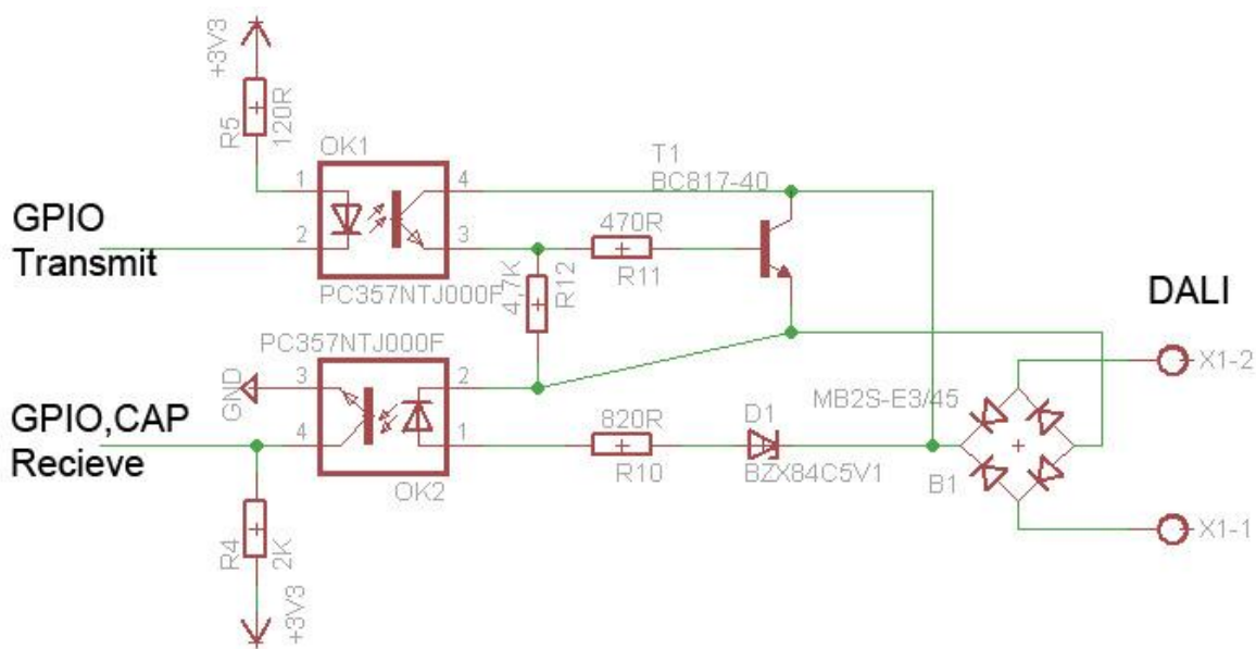
Obrázok 6.3 Zapojenie optickej izolácie DALI
