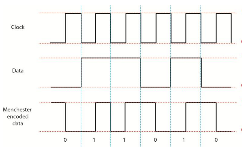
Obrázok 4.3 Manchesterské kódovanie
