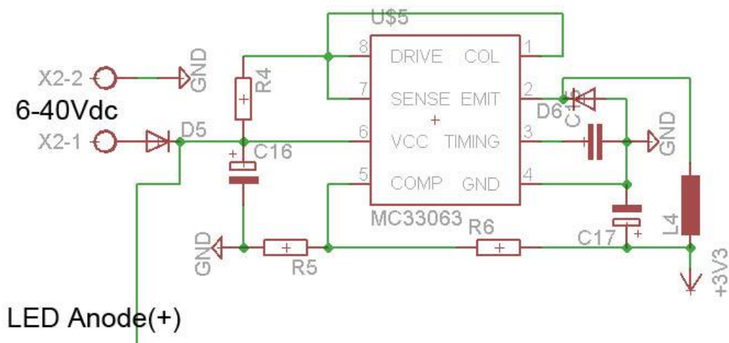
Obrázok 6.2 Regulátor napätia
