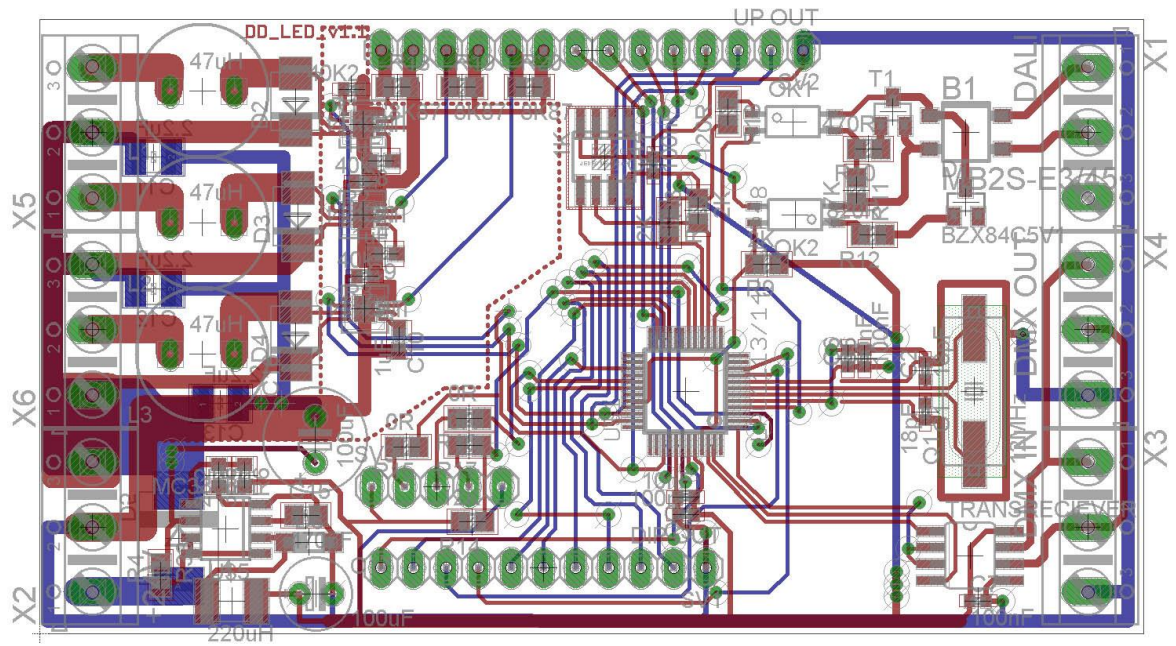
Obrázok D.2 Schéma spodného plošného spoja
