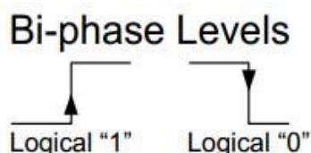
Obrázok 4.2 Bi-fázové kódovanie bitov[5]
