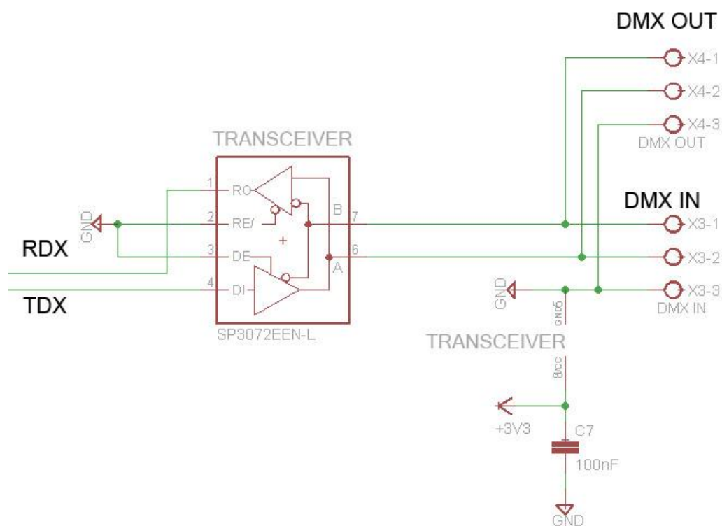
Obrázok 6.5 Zapojenie DMX
