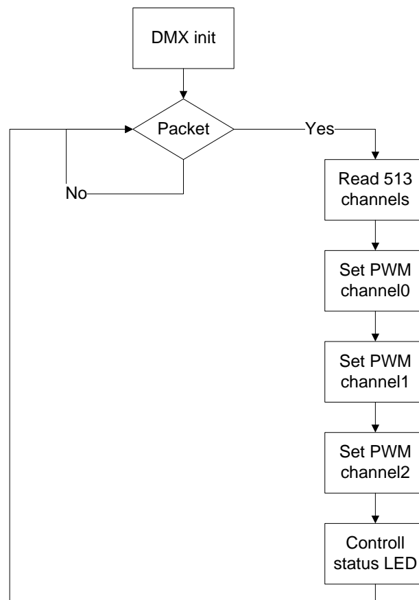
Obrázok 7.2 Flowchart DMX
