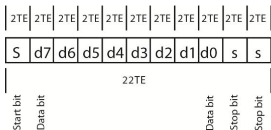
Obrázok 4.5 Formát Backward Paketu DALI[5]
