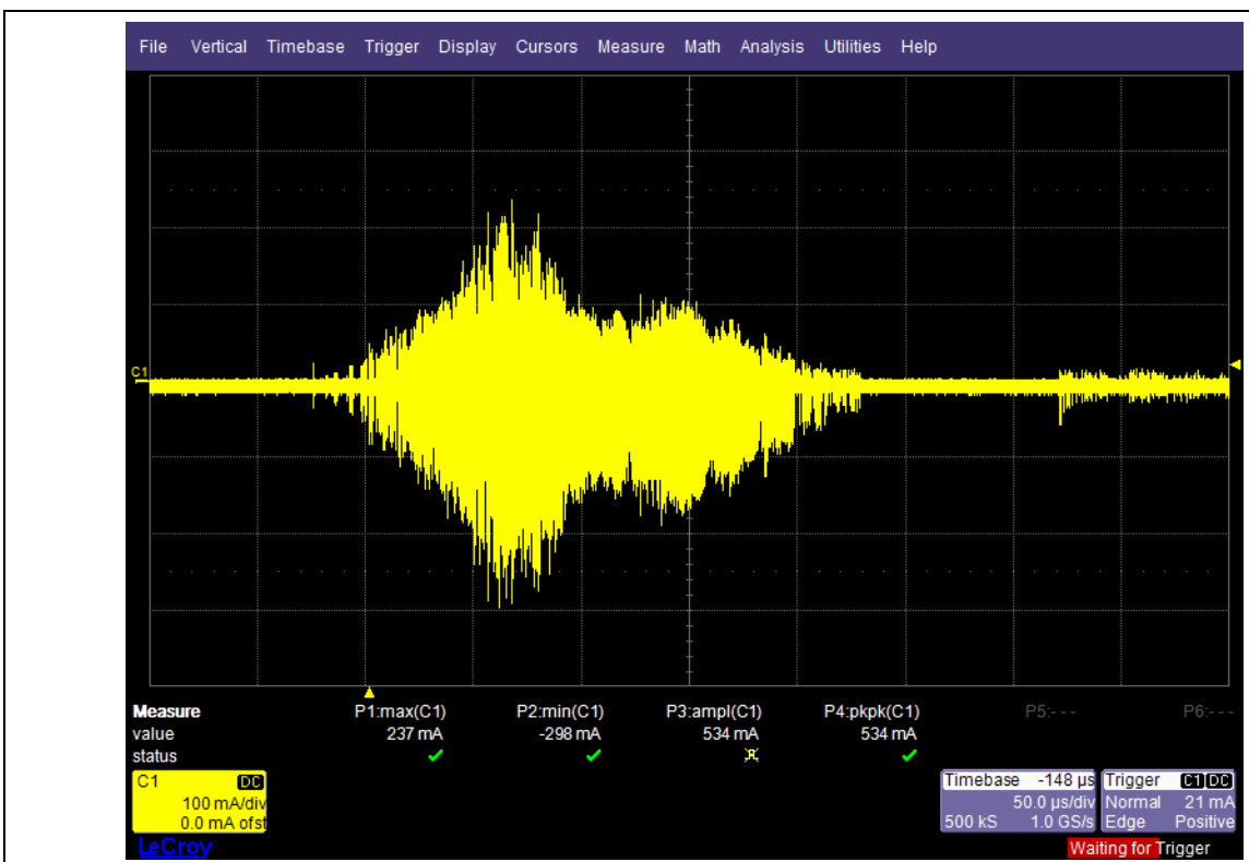
Obr 18. Průběh proudu cívkou AML při odpojení napájení
