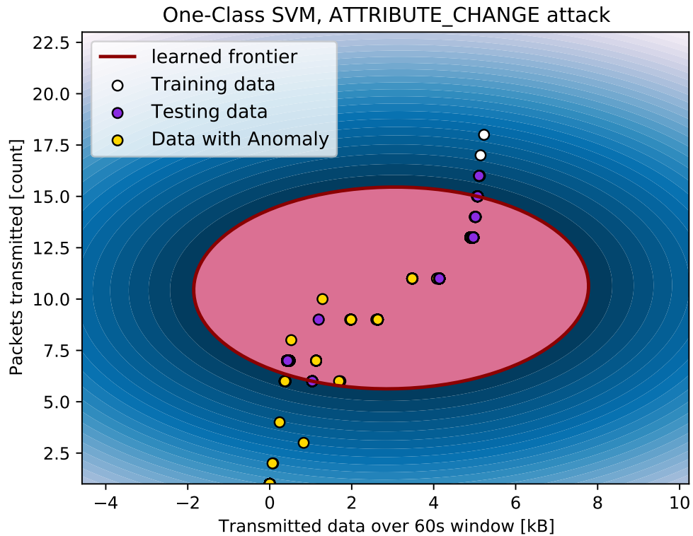
Obr. 5.14: One-Class SVM, útok Modify parameter na komunikáciu (RTU->HMI)
