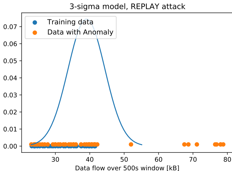
Obr. 5.8: Three-Sigma, útok Replay na komunikáciu (RTU->HMI)
