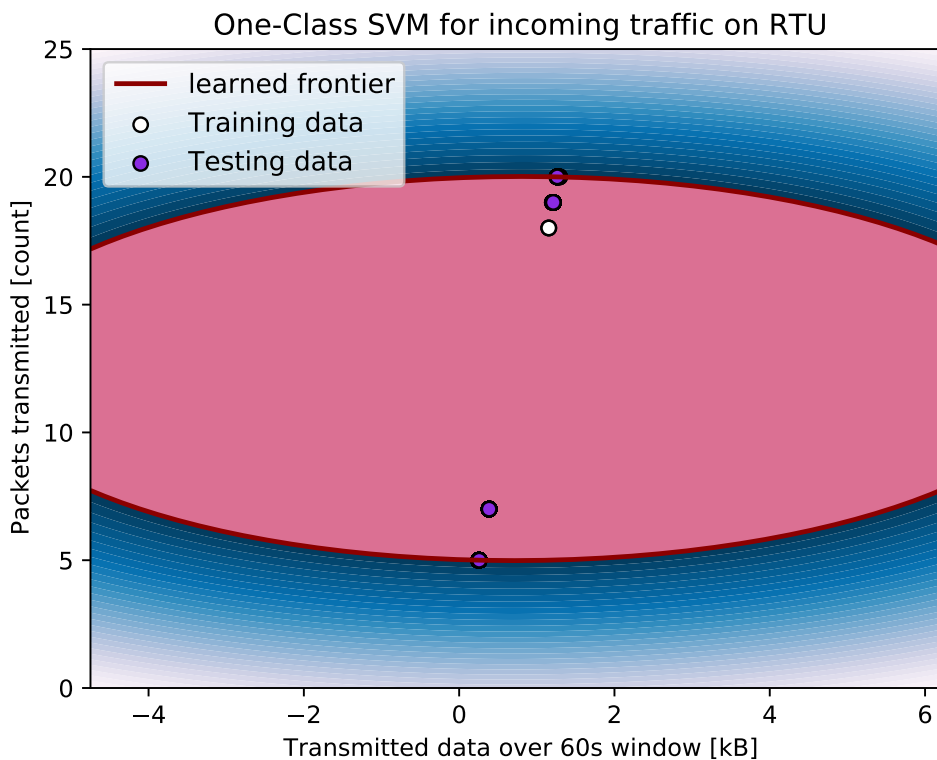
Obr. 5.7: One-Class SVM na strane prichodzej komunikácie na zariadenie HMI
